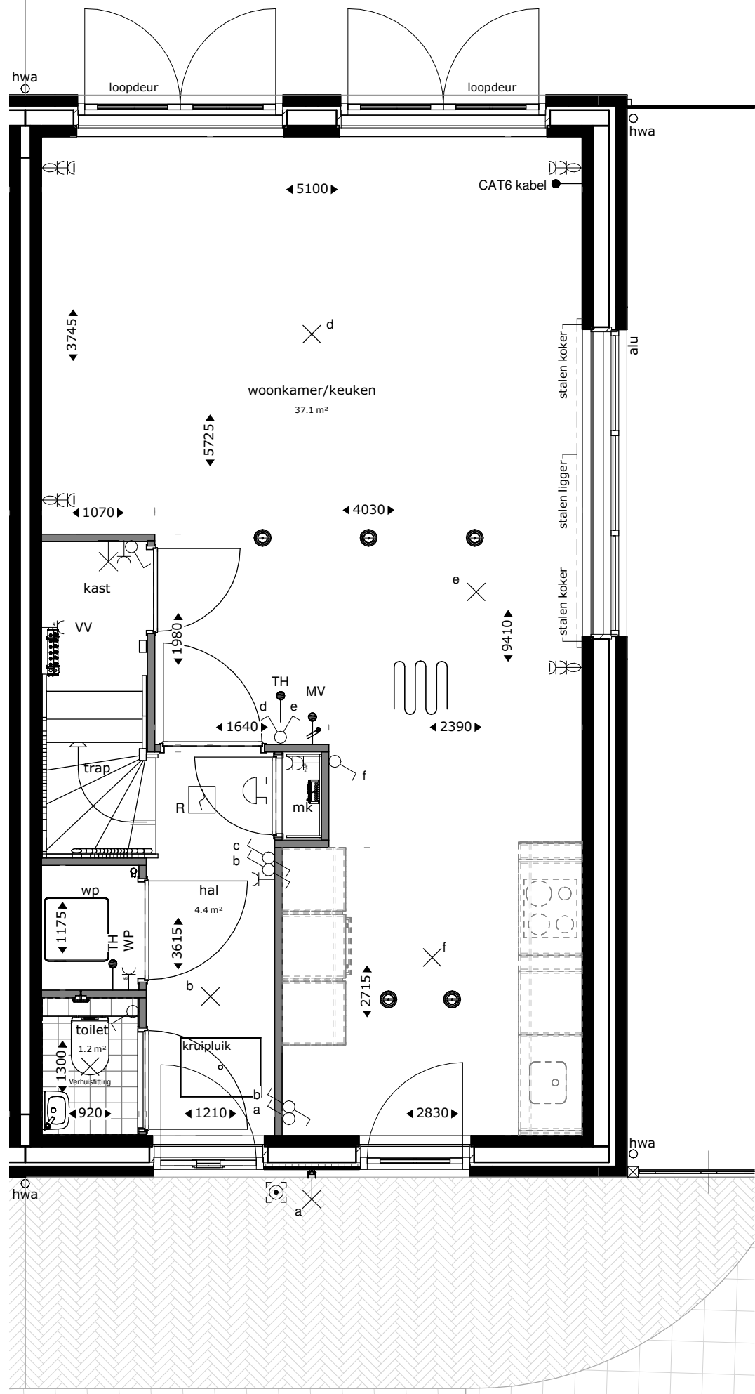
begane grond
