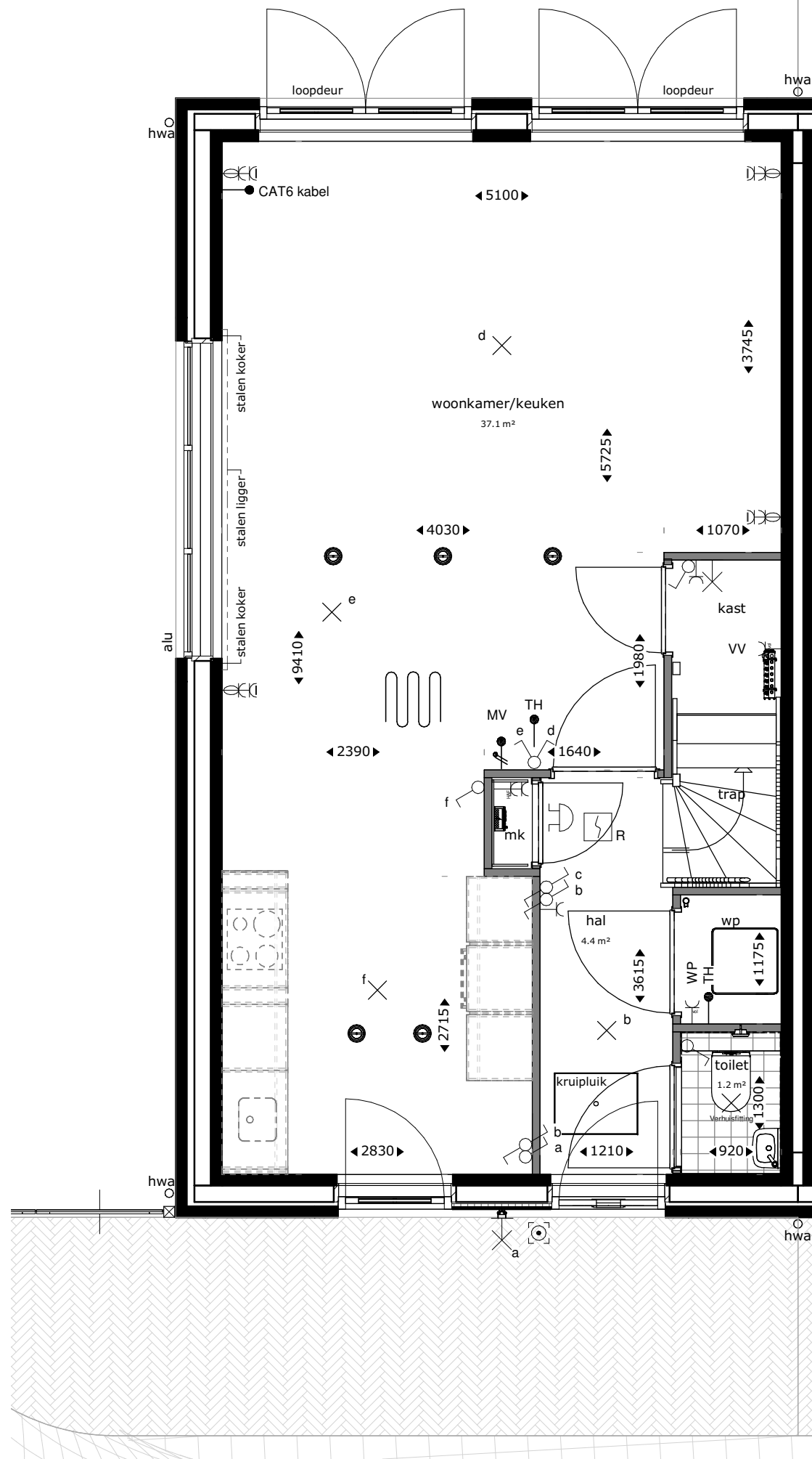
begane grond
