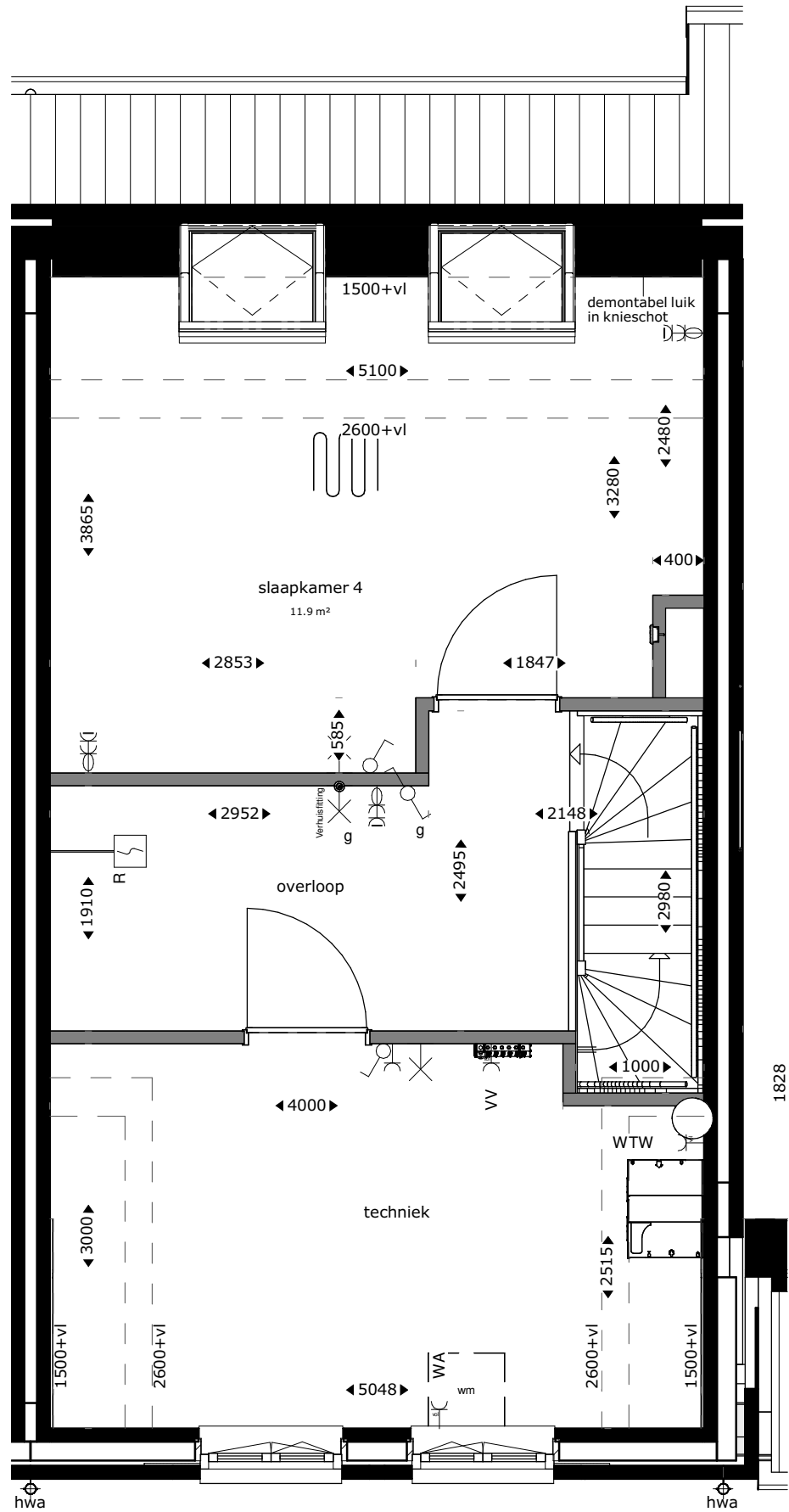
tweede verdieping
