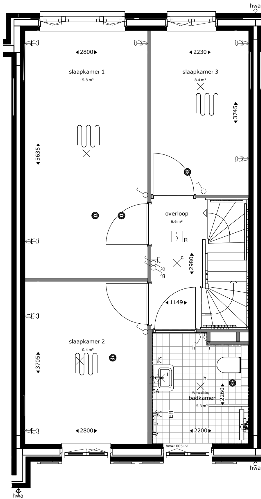
eerste verdieping
