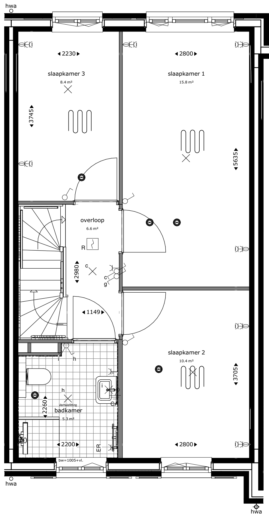
eerste verdieping
