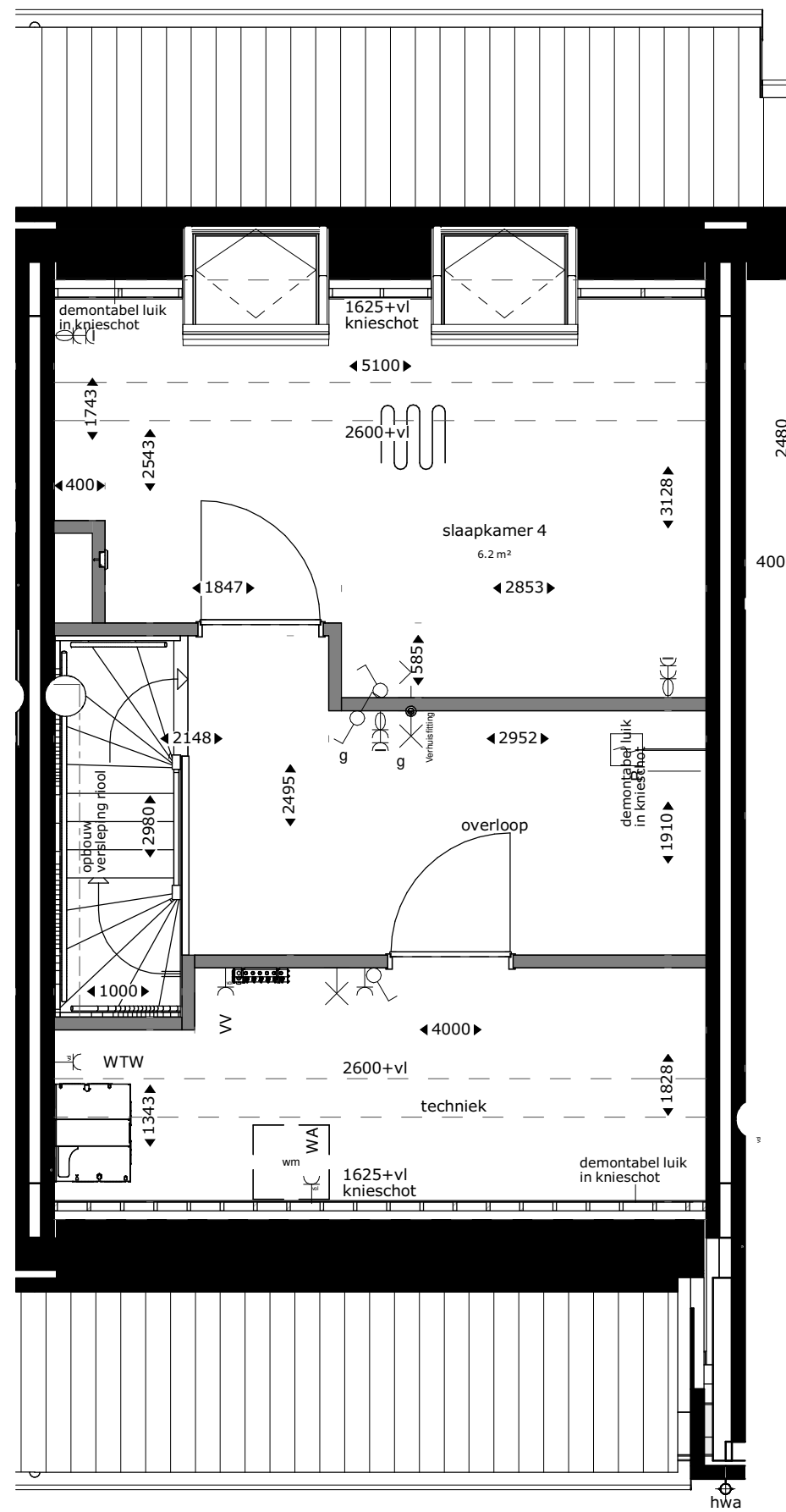
tweede verdieping
