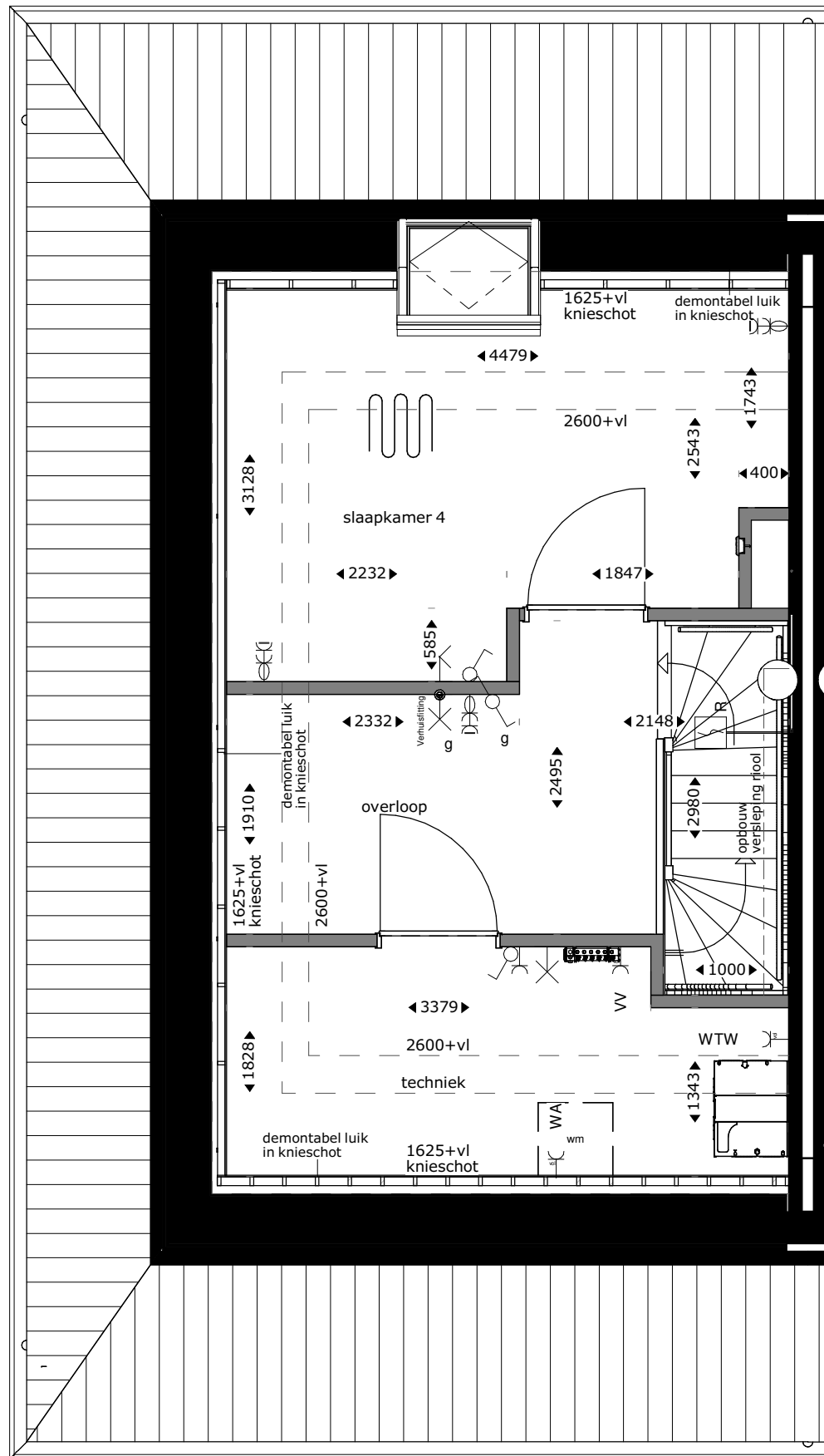
tweede verdieping
