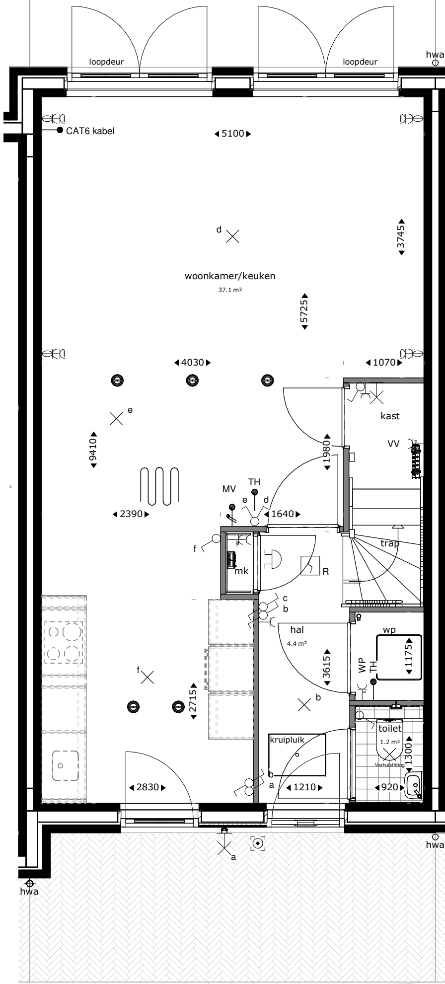
begane grond
