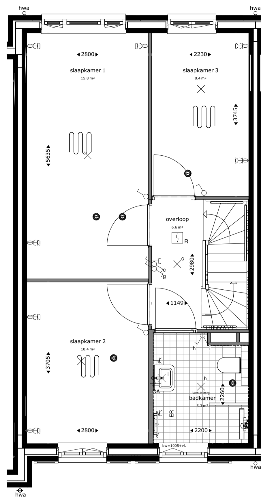
eerste verdieping
