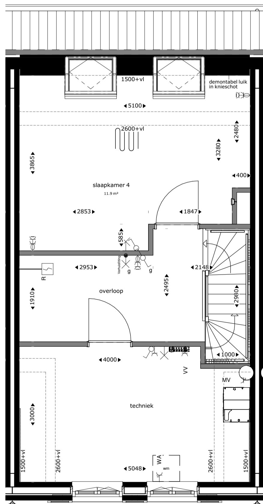
tweede verdieping
