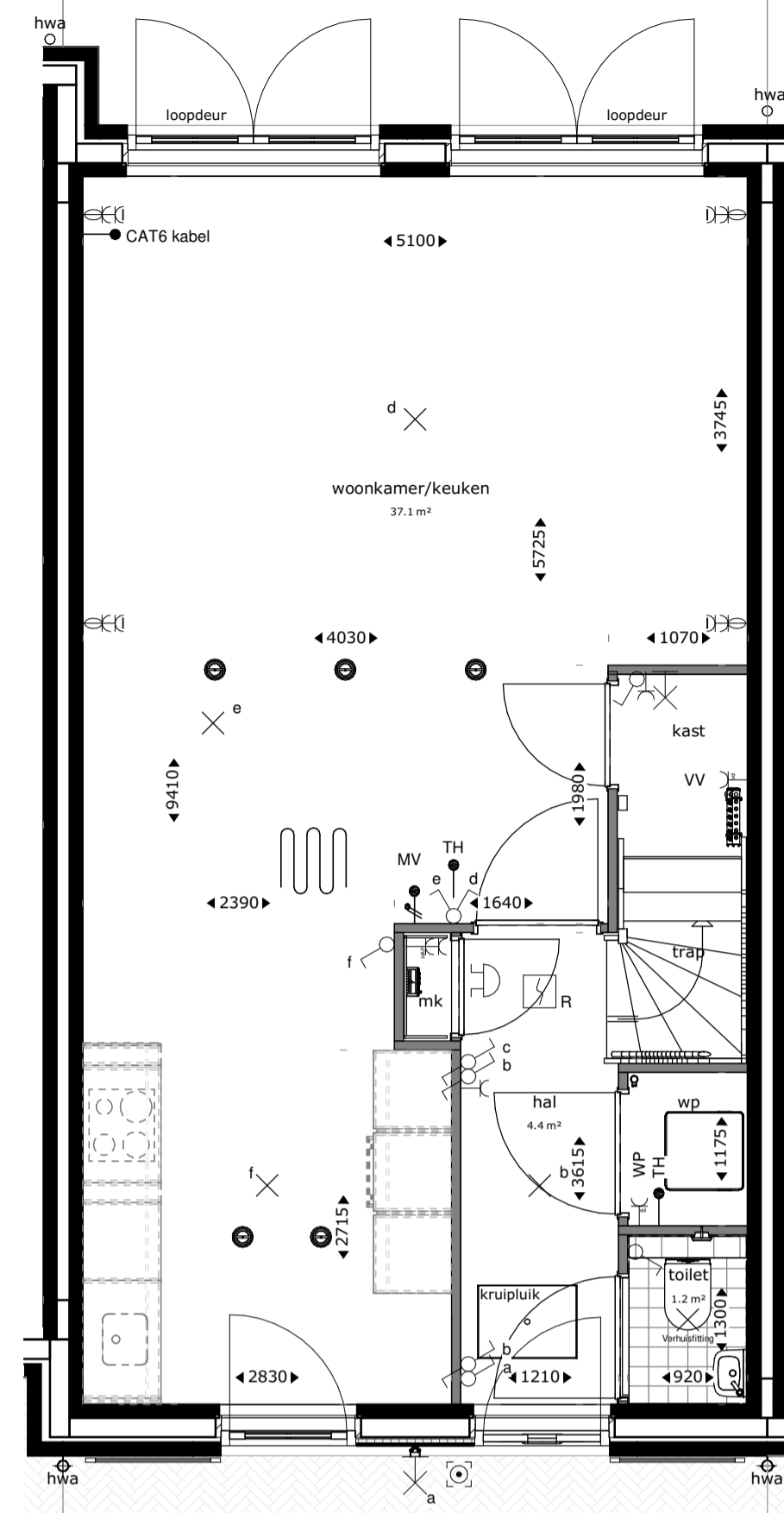
begane grond
