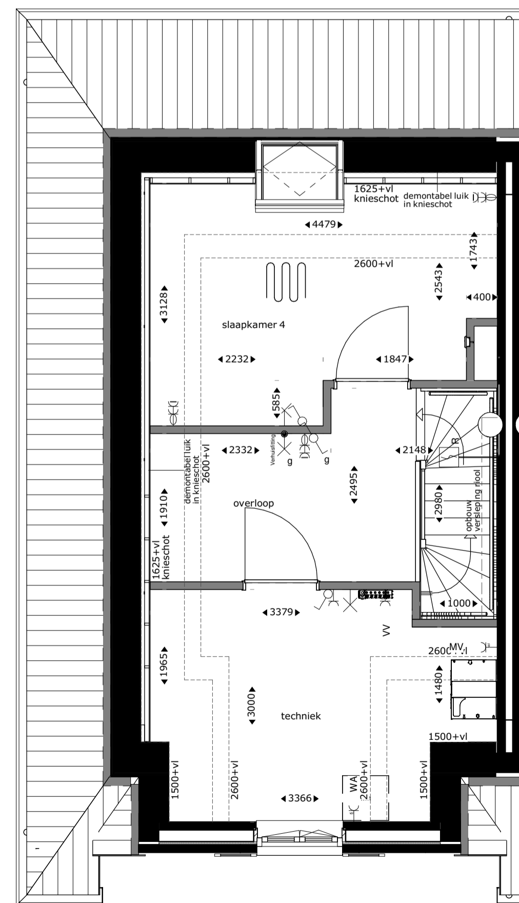
tweede verdieping
