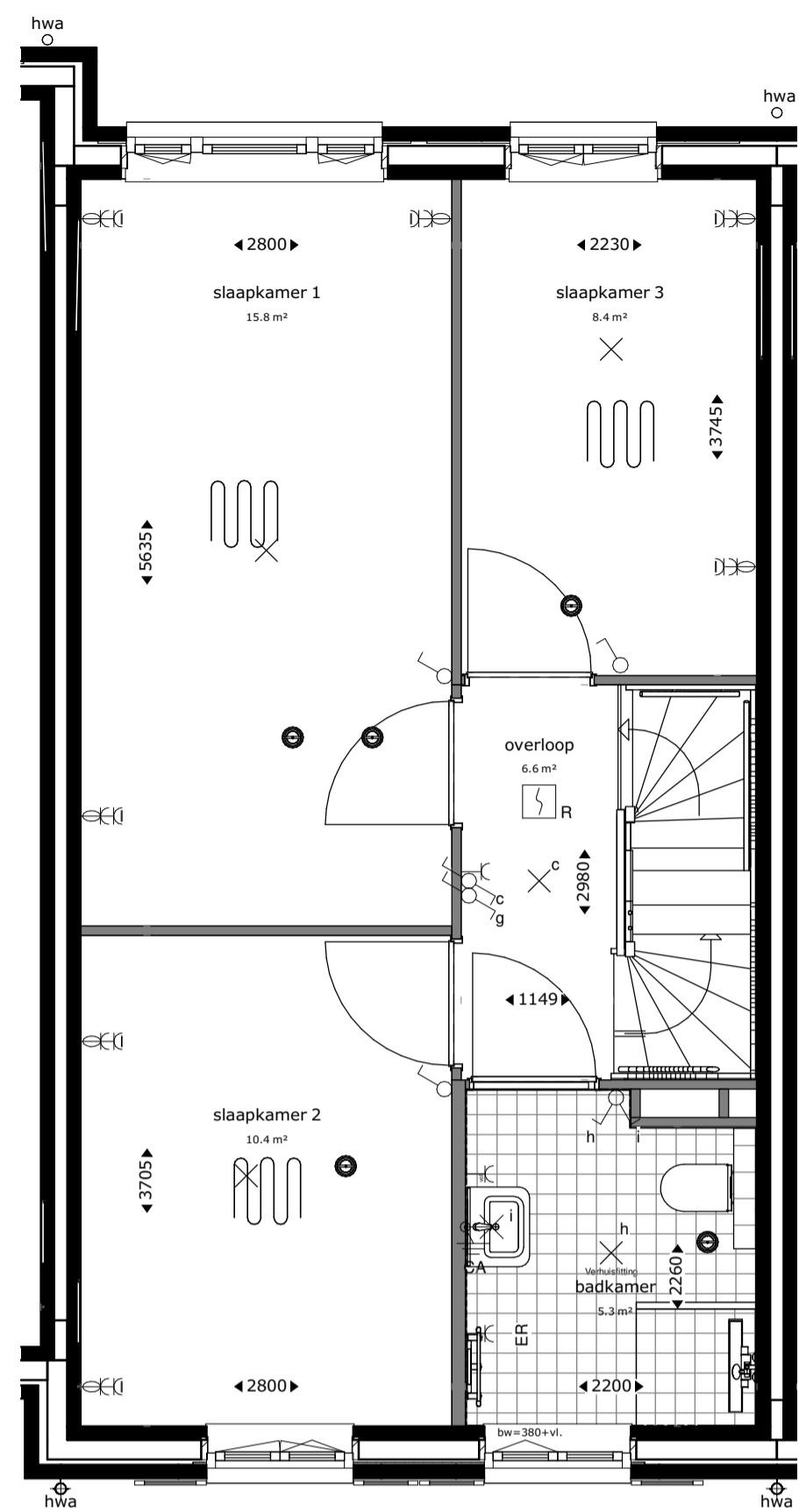
eerste verdieping
