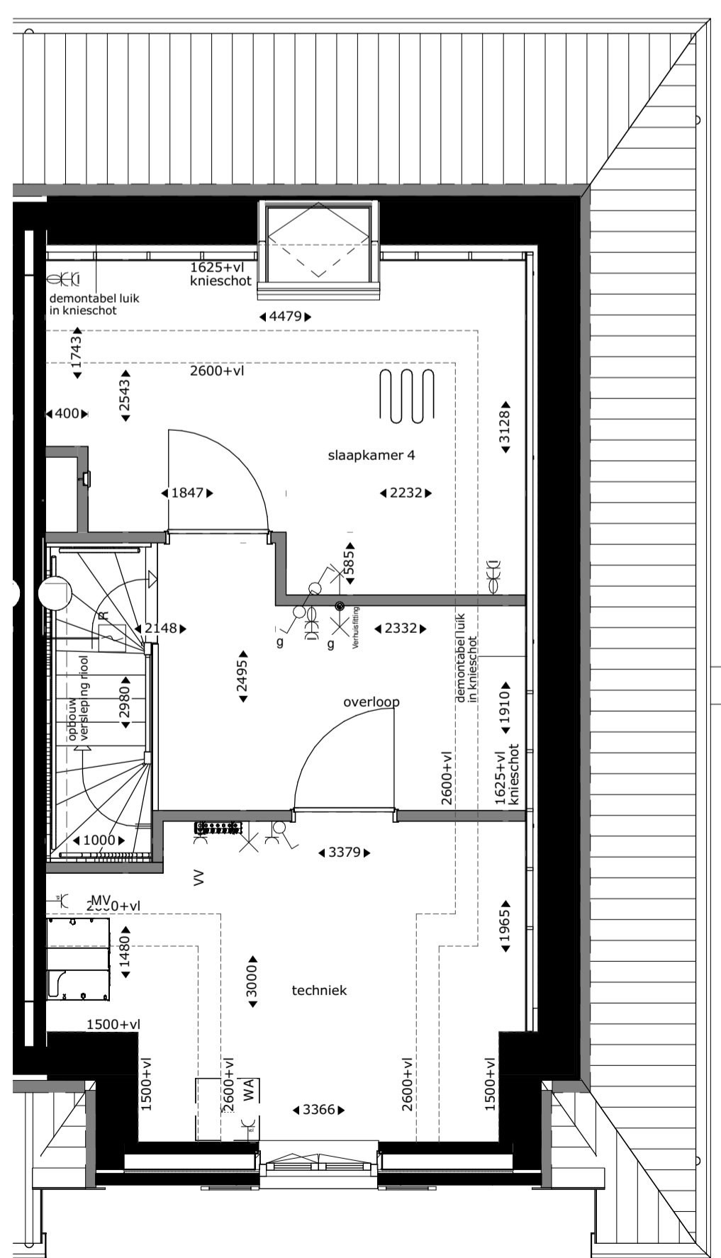
tweede verdieping
