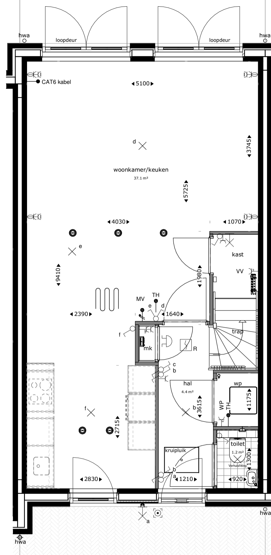
begane grond
