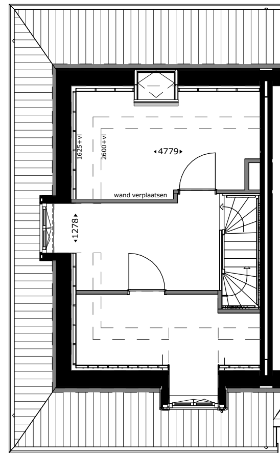
Dakkapel zijgevel (vergunningplichtig) getekend: bwnr 03
