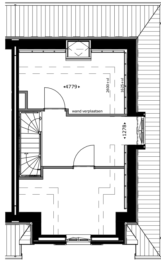
Dakkapel zijgevel (vergunningplichtig) getekend: bwnr 04
