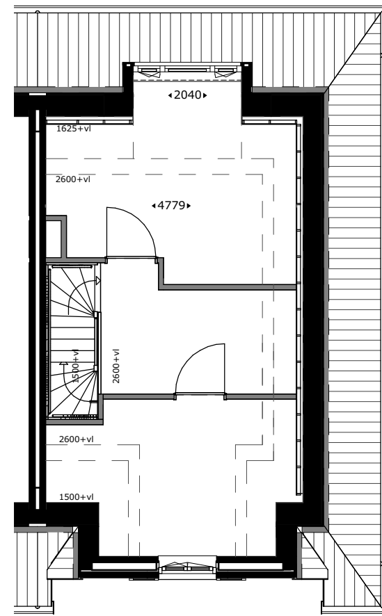
Dakkapel achtergevel getekend: bwnr 04
