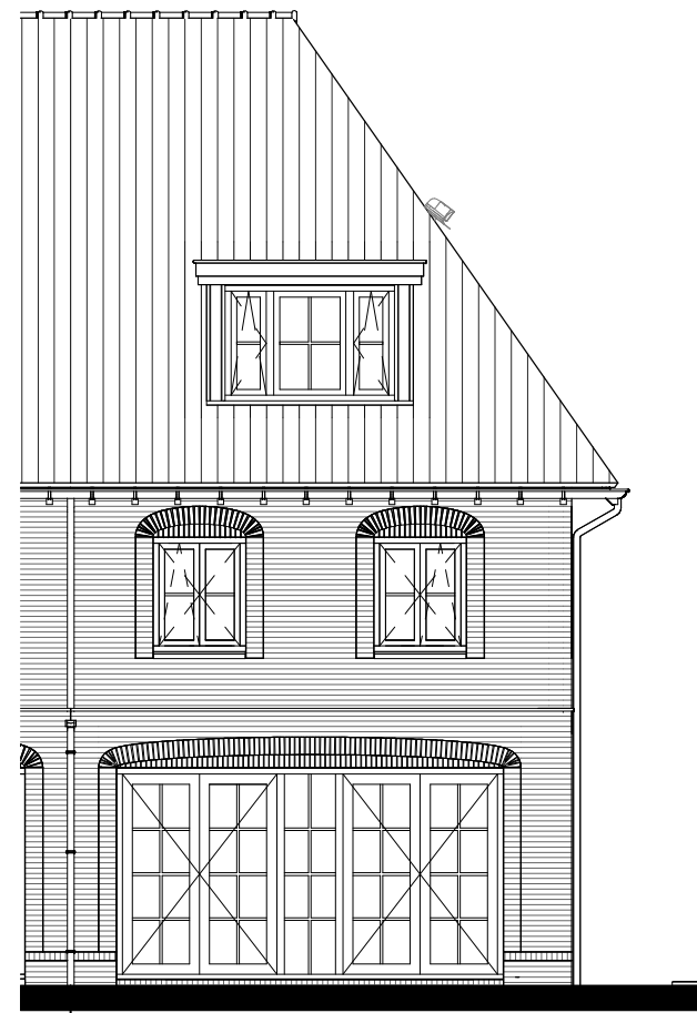
Vergrootte pul getekend: bwnr 03 gespiegeld: bwnr 04
