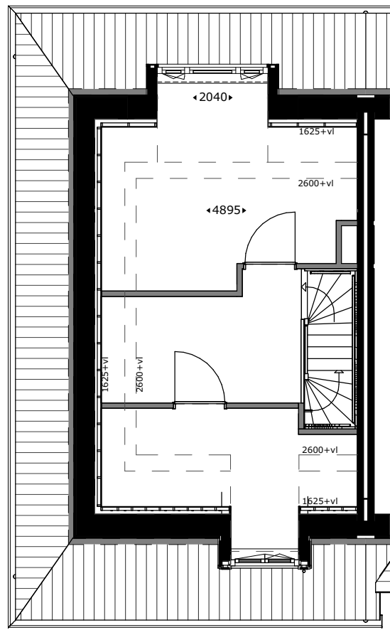
Dakkapel achtergevel getekend: bwnr 03
