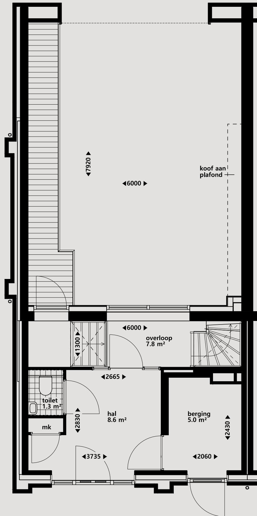
BEGANE GROND NIET OP SCHAAL
