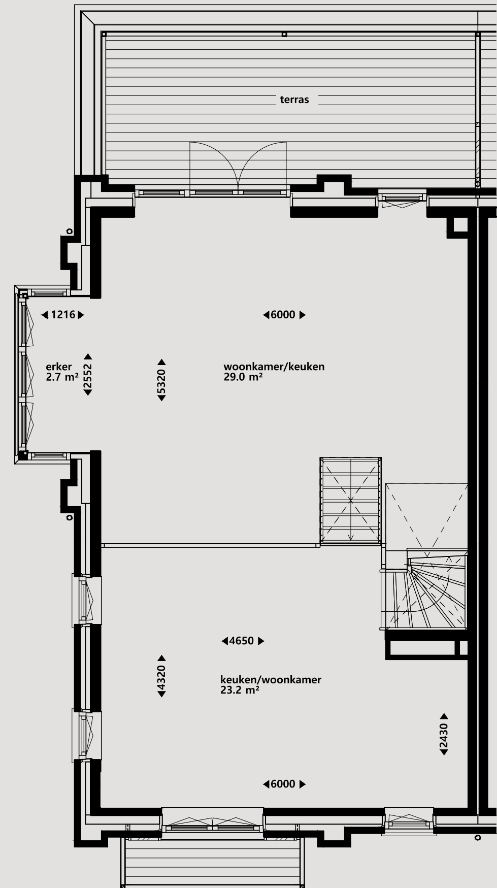
1 e VERDIEPING NIET OP SCHAAL
