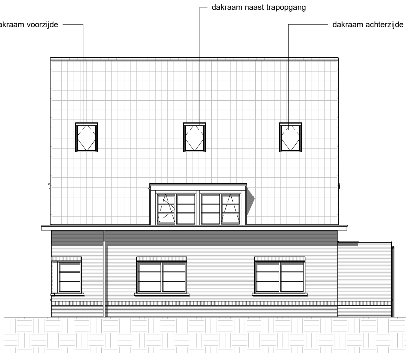
rechtter zijgevel
