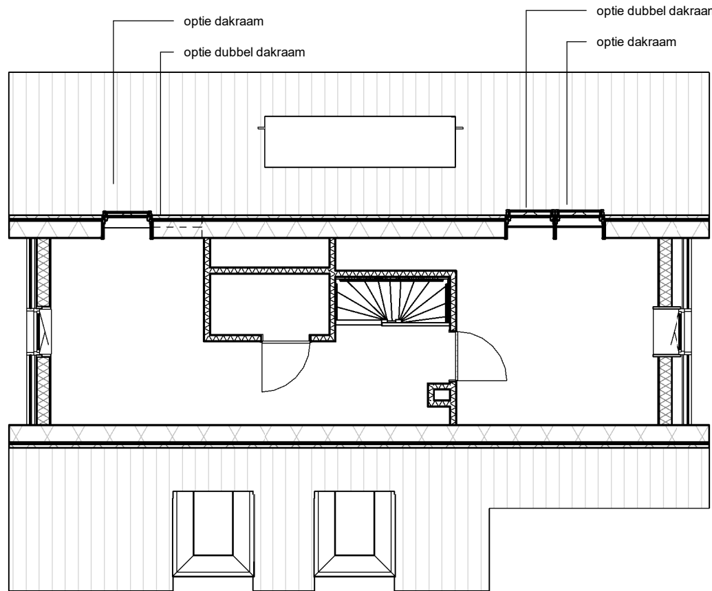
2e verdieping
