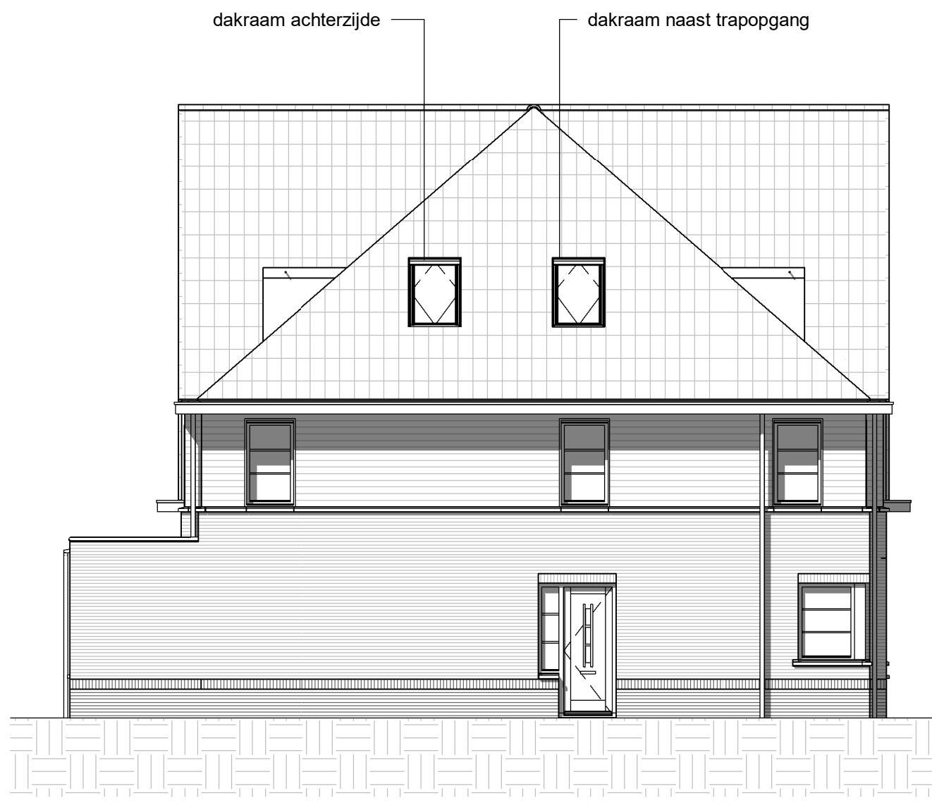
zijgevel
