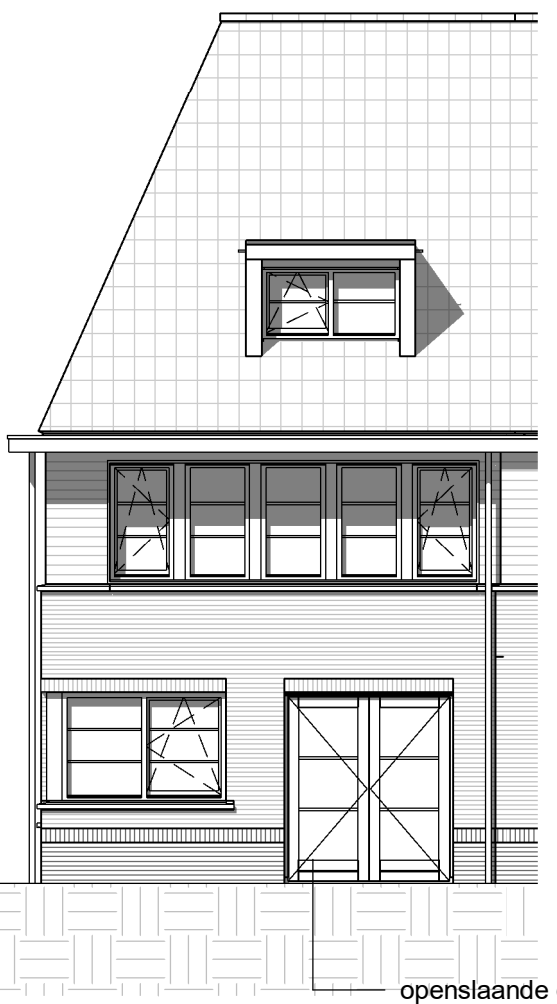
voorgevel
