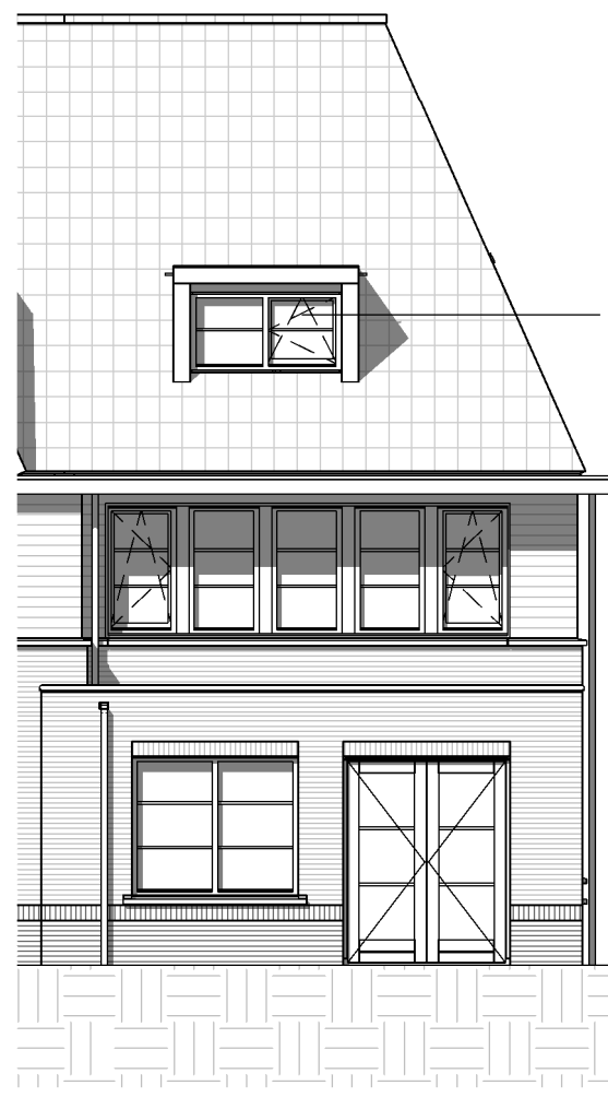
achtergevel
