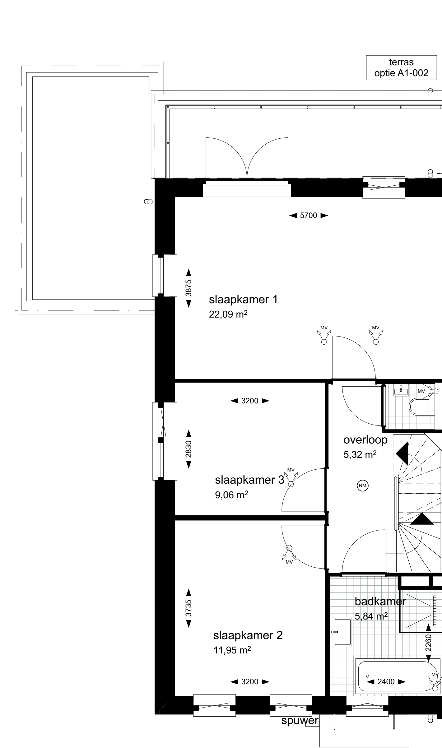
1:50 01 eerste verdieping
