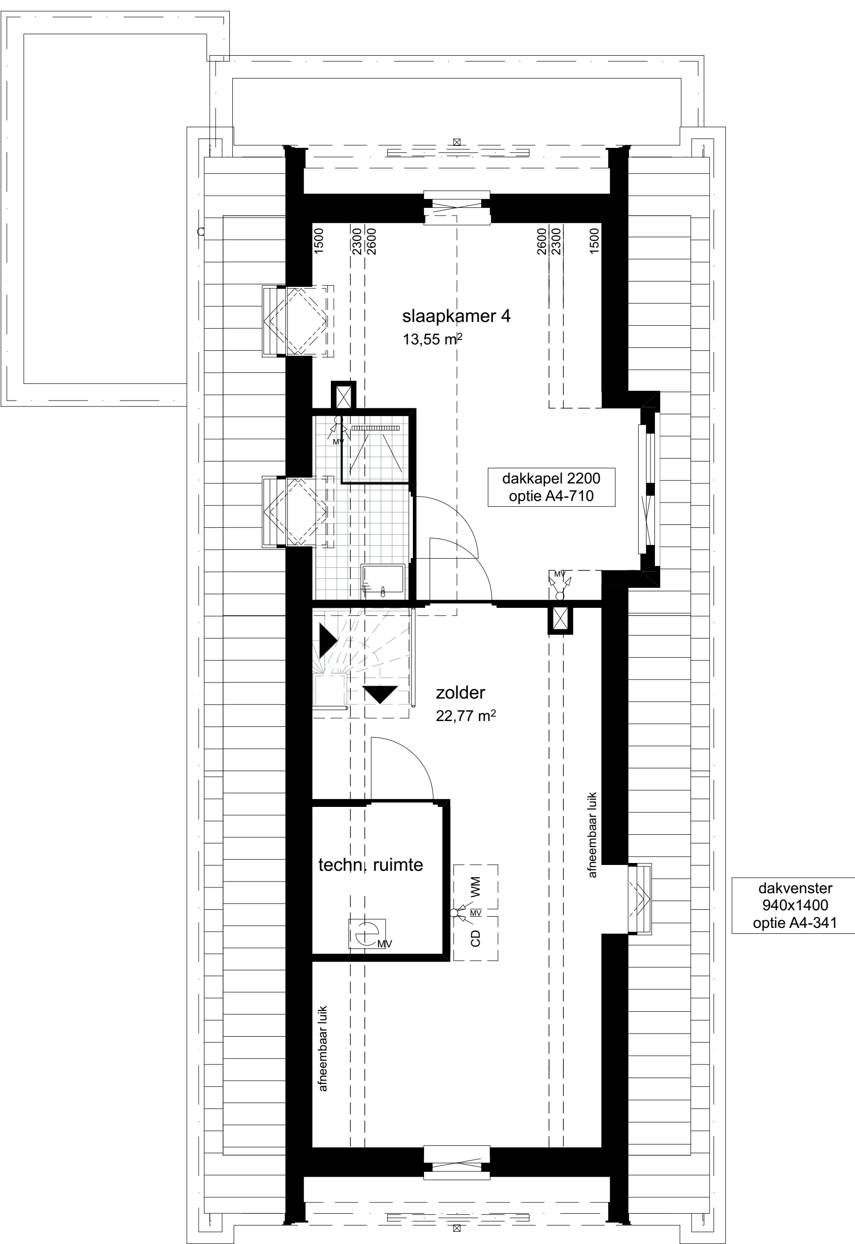
1:50 02 tweede verdieping
