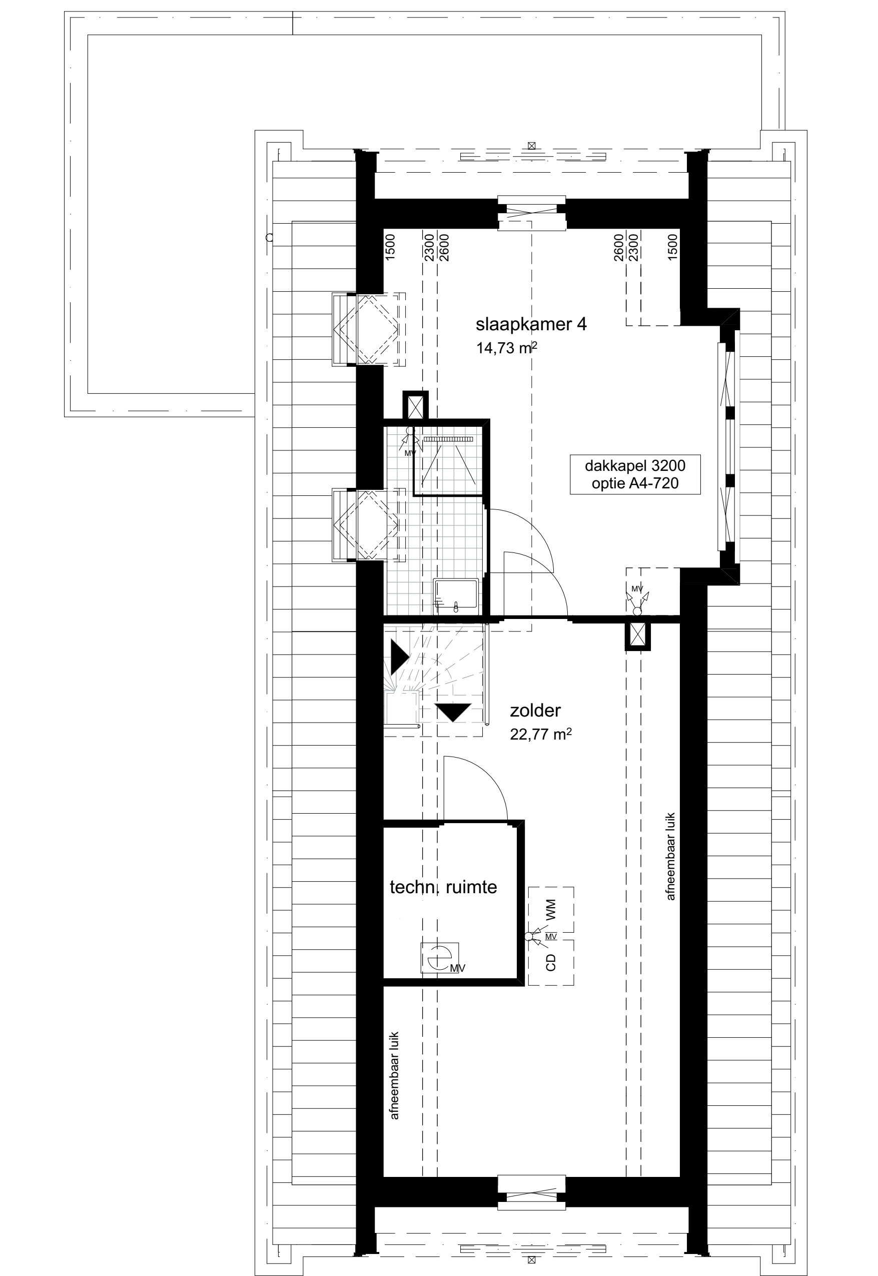
1:50 02 tweede verdieping
