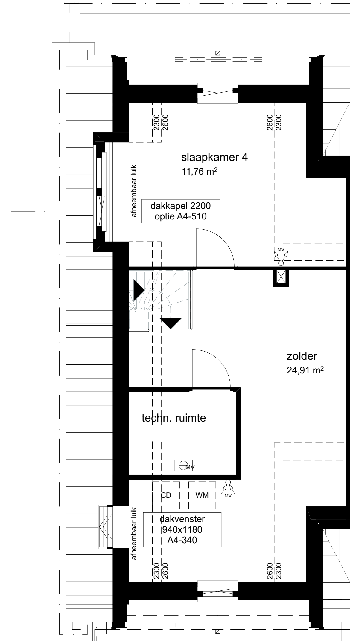
1:50 02 tweede verdieping
