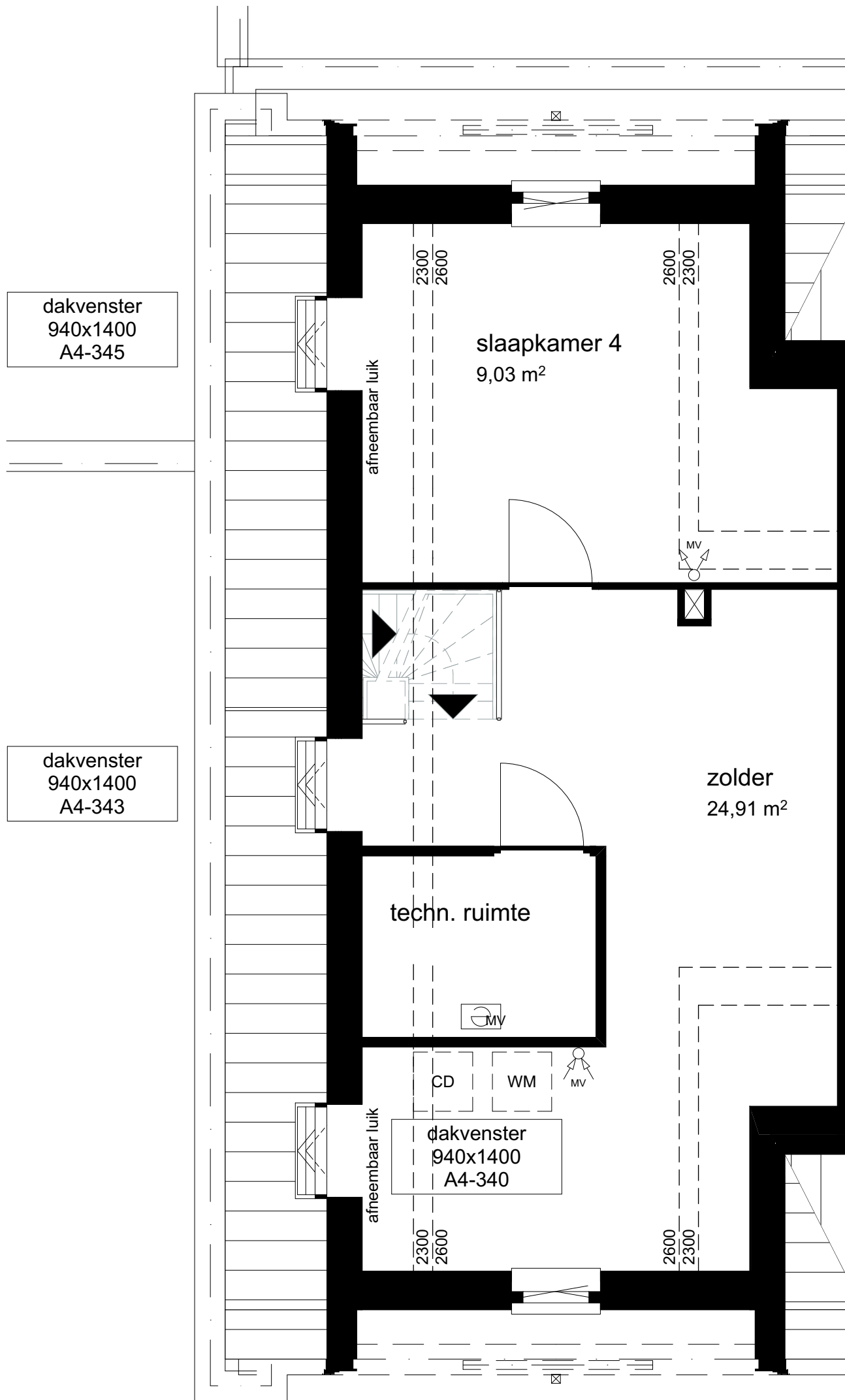
1:50 02 tweede verdieping
