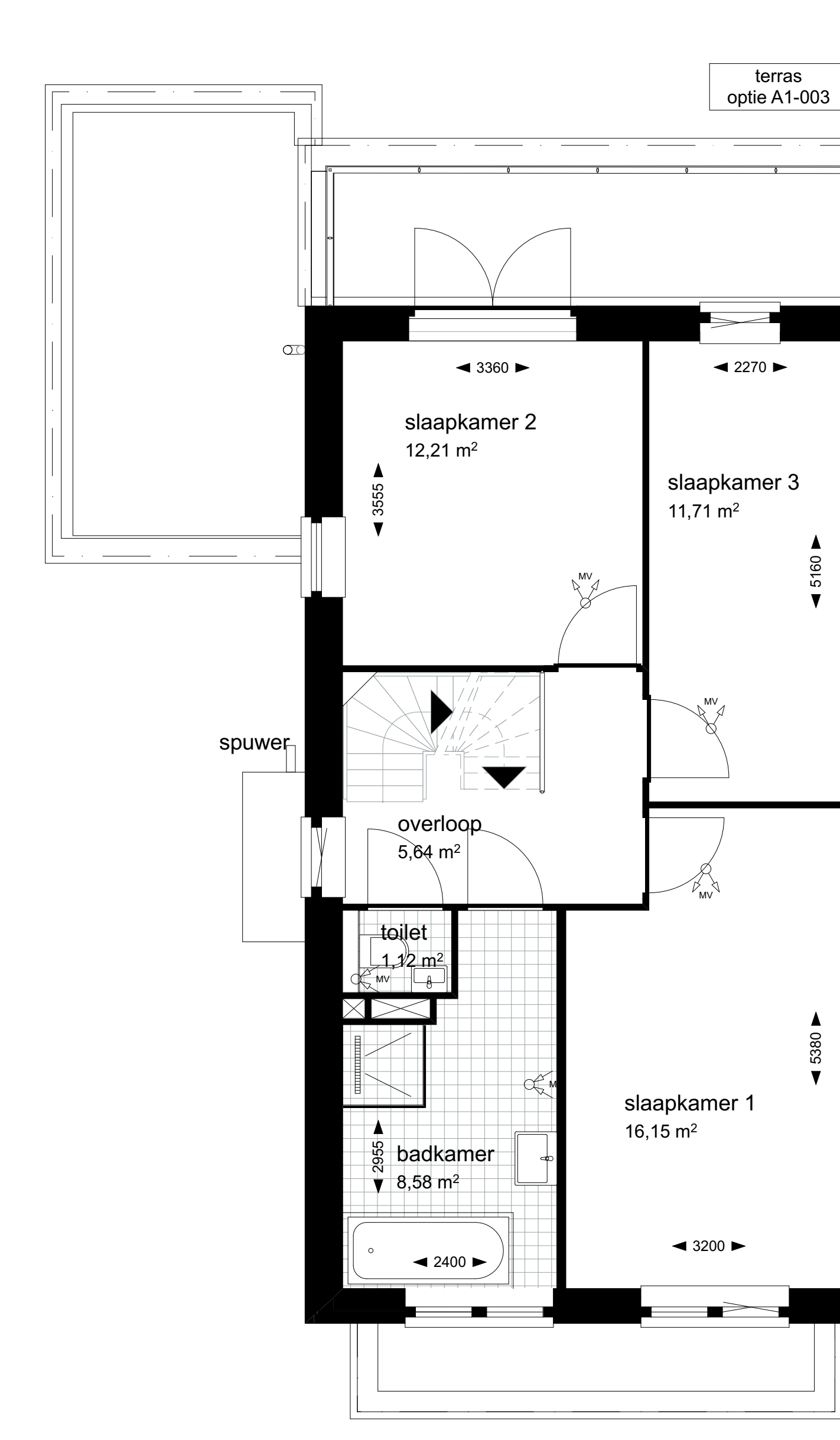
1:50 01 eerste verdieping
