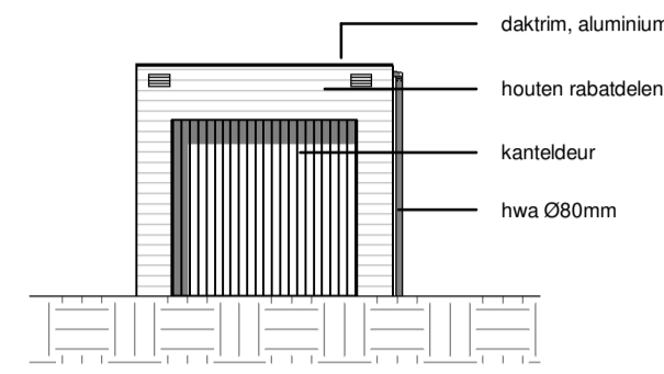
voorgevel berging type A
