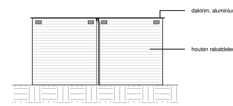
achtergevel dubbele berging
