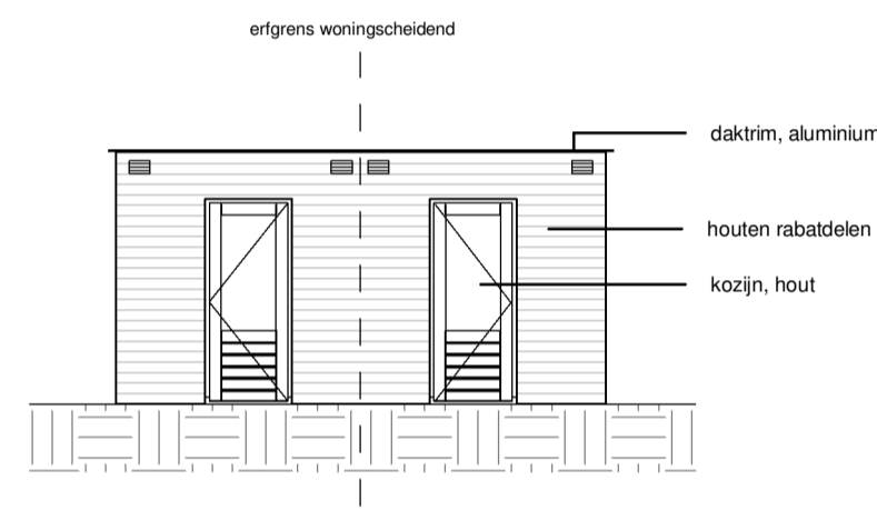
voorgevel dubbele berging type B
