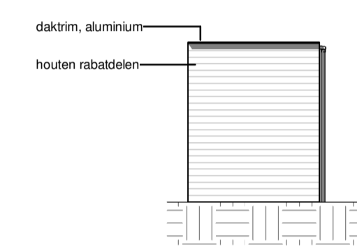
rechter zijgevel dubbele berging
