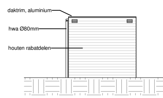
achtergevel berging
