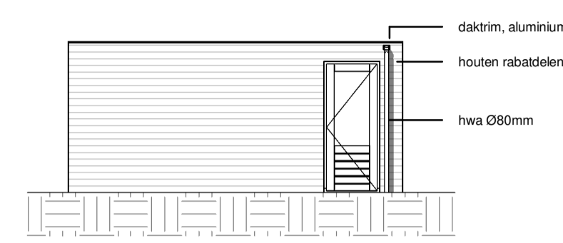
rechter zijgevel
