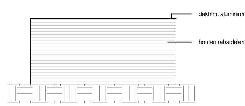
linker zijgevel
