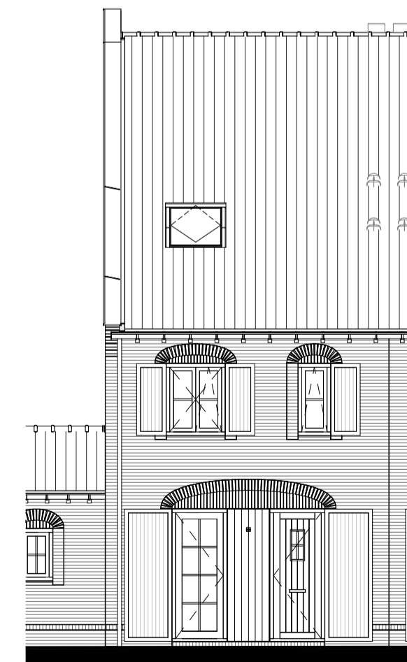
Dakraam voorgevel (vergunningplichtig) getekend : bwnr 21 gespiegeld: bwnr 22
