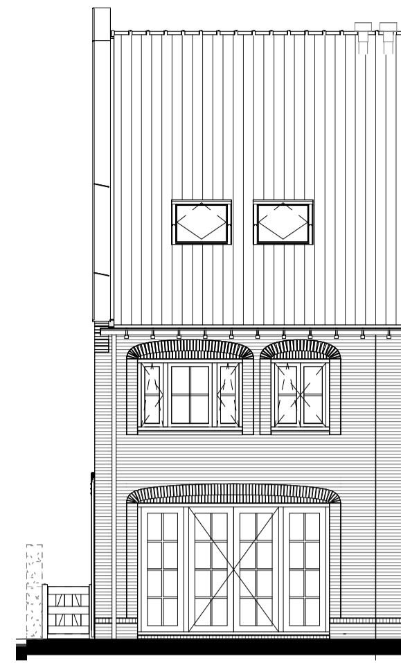
Vergrootte pui. getekend : bwnr 22
