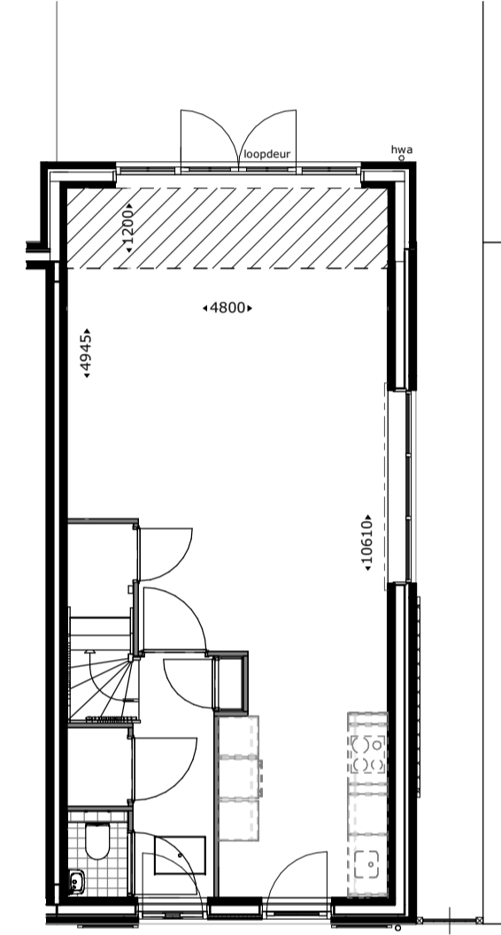
Uitbouw 1200mm. getekend: bwnr 22
