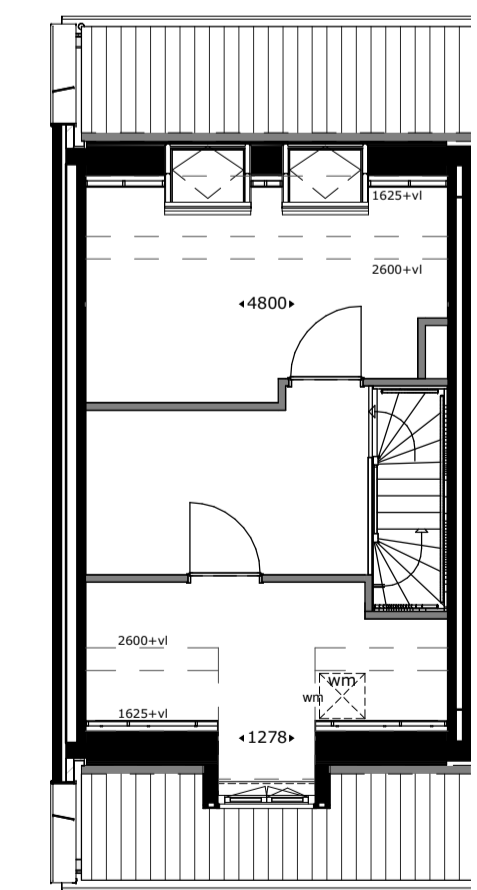
Dakkapel voorgevel (vergunningplichtig) getekend : bwnr 21 gespiegeld: bwnr 22
