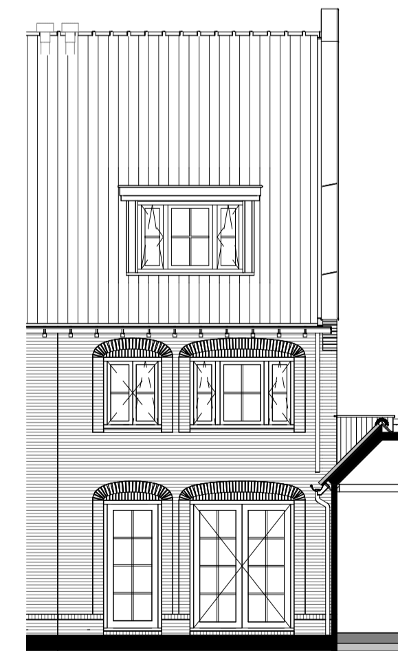
Dakkapel achtergevel getekend : bwnr 21 gespiegeld: bwnr 22
