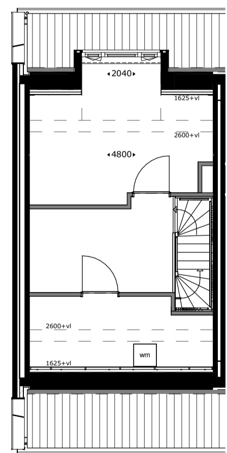
Dakkapel achtergevel getekend: bwnr 21 gespiegeld: bwnr 22
