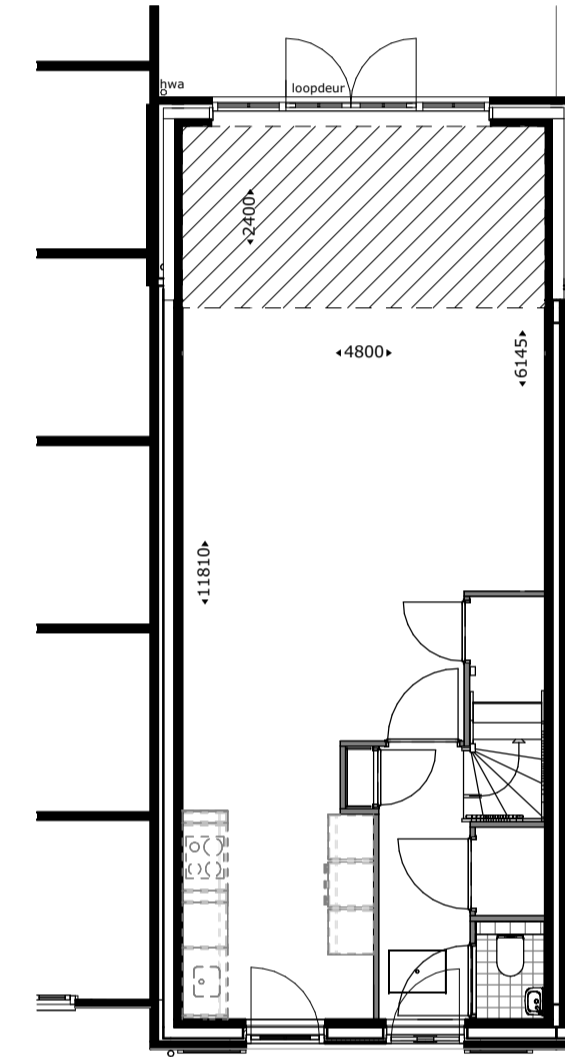
Uitbouw 2400mm. getekend: bwnr 21
