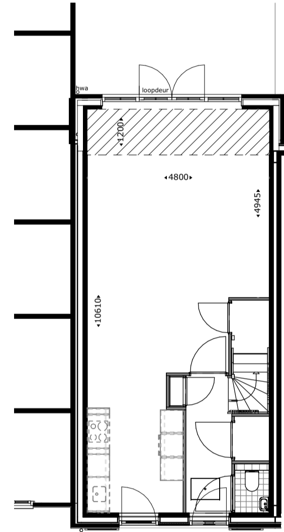
Uitbouw 1200mm. getekend: bwnr 21
