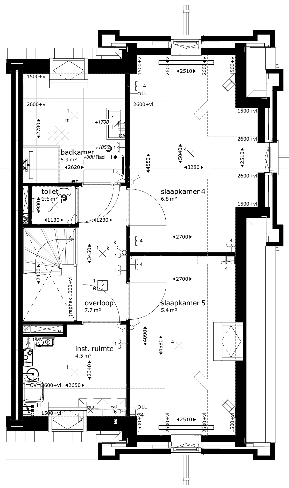
derde verdieping
