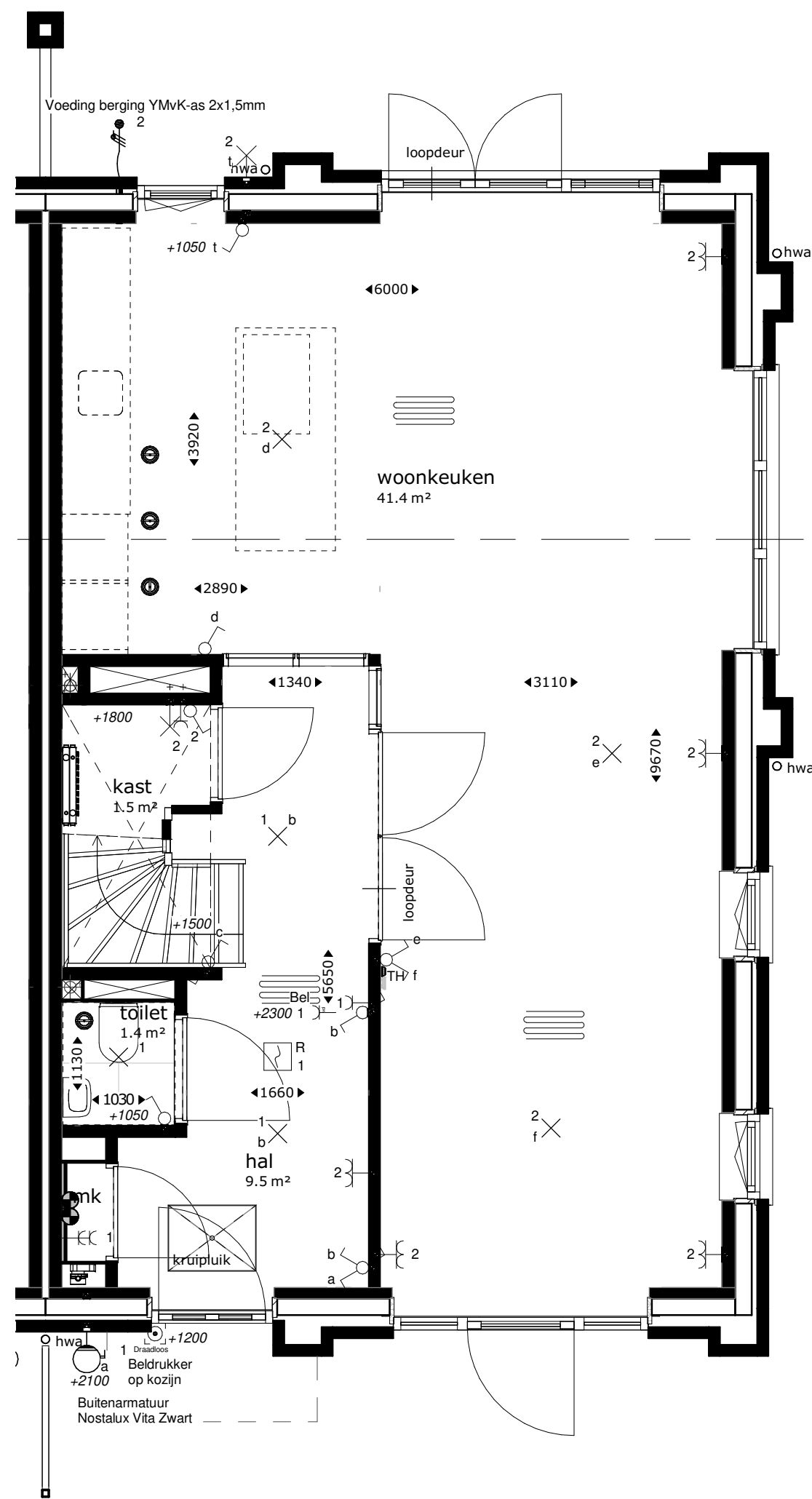
begane grond
