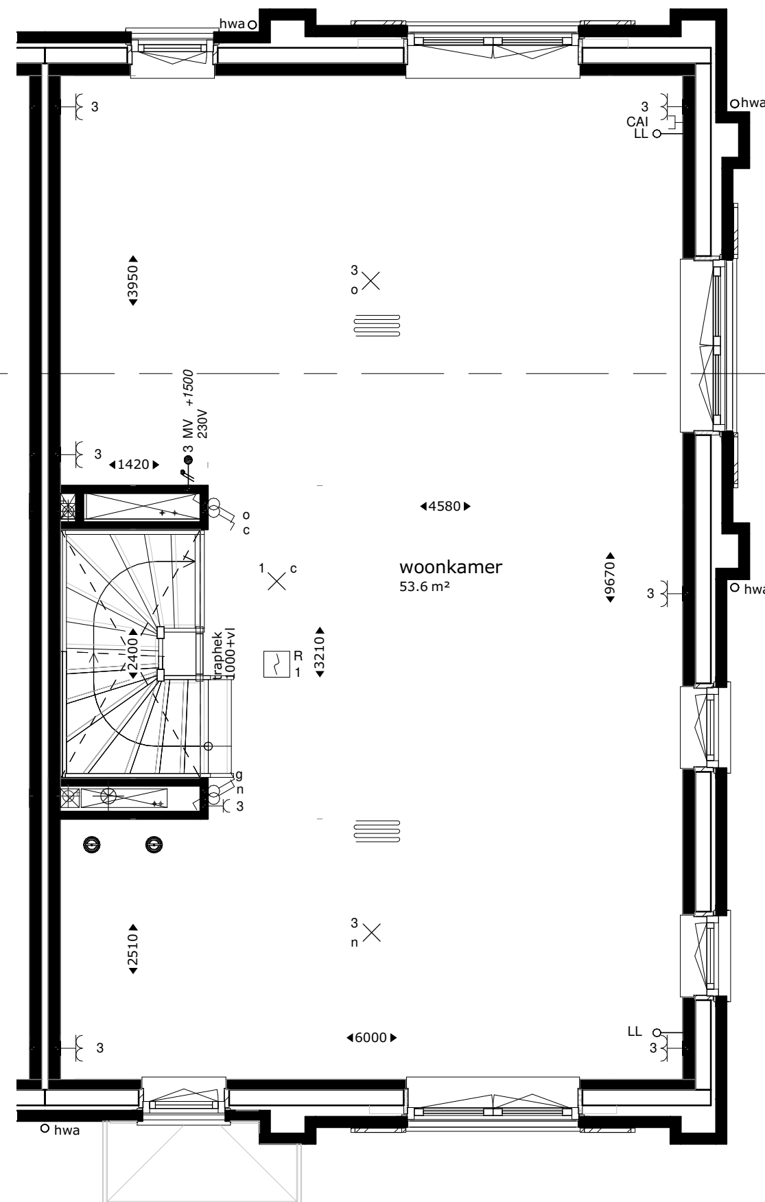
eerste verdieping
