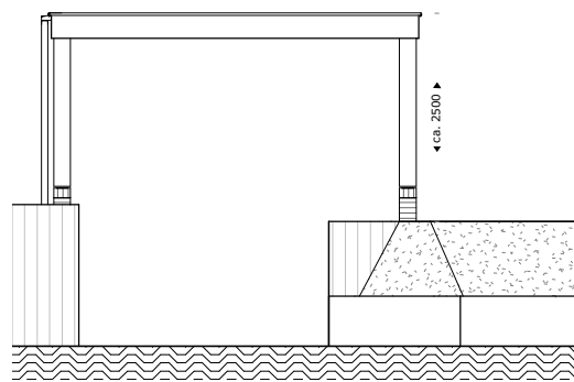
boothuis achtergevel
