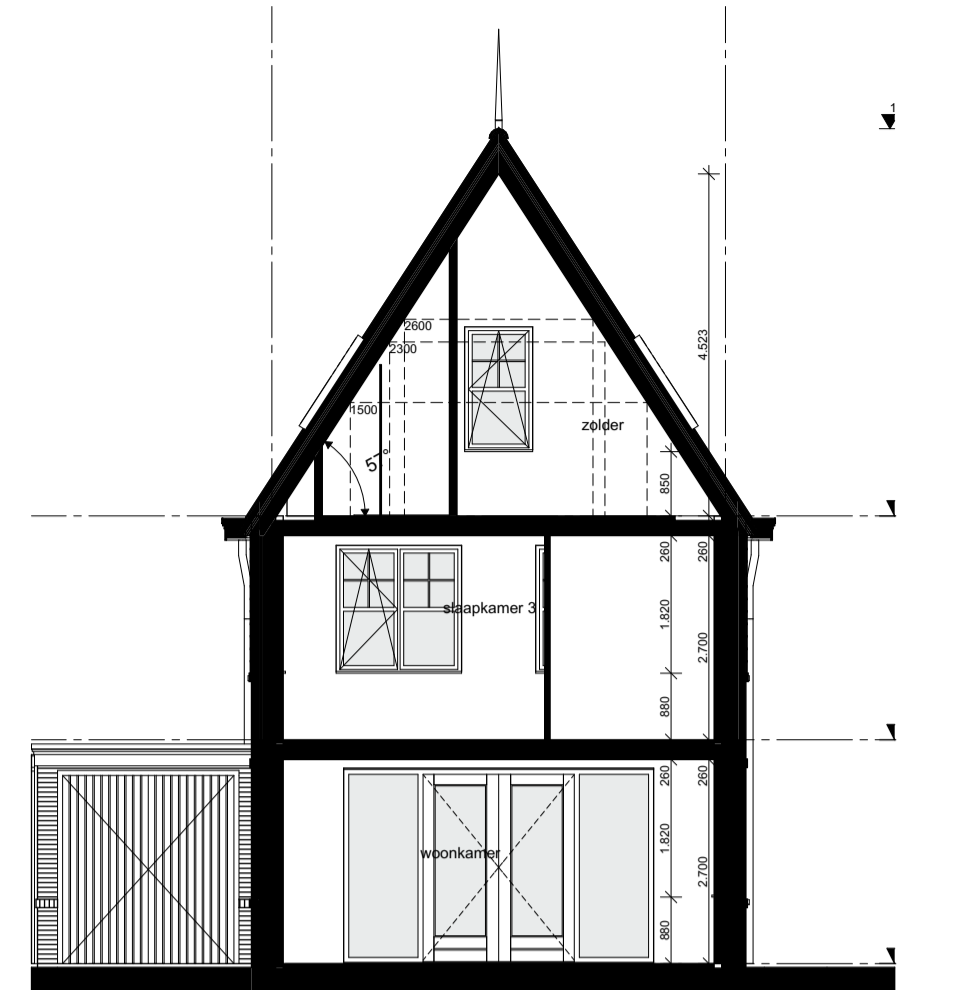
1:100 Doorsnede A-A
