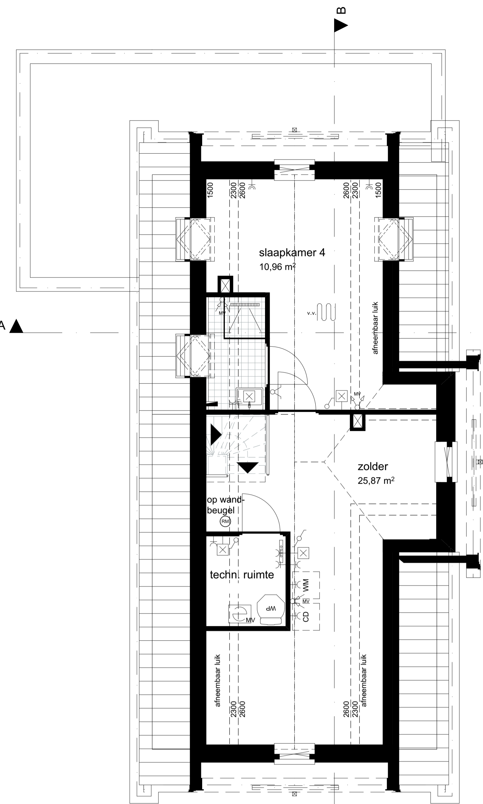
1:50 02 tweede verdieping
