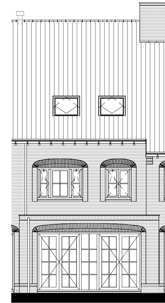
Uitbouw 3200mm getekend: bwnr 23,28 gepegeld: bwnr 27
