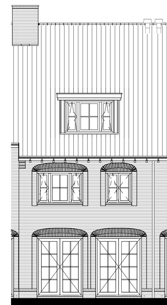
Dakkapel achtergevel getekend: bwnr 28 gepegeld: bwnr 29
