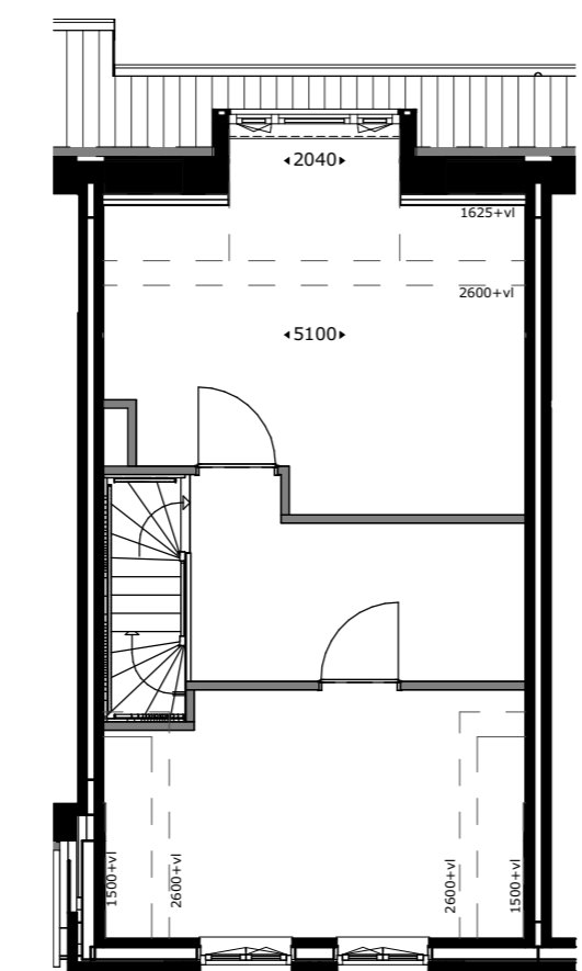
Dakkapel achtergevel getekend: bwnr 23 gepegeld: bwnr 29
