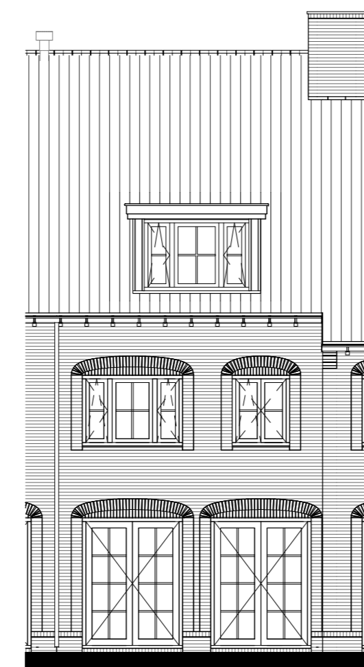
Dakkapel achtergevel getekend: bwnr 23,28 gepegeld: bwnr 29
