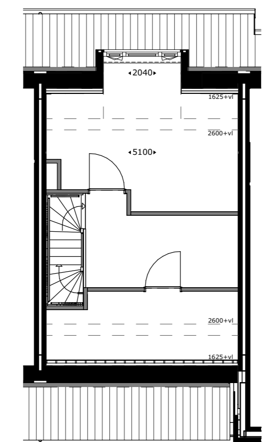
Dakkapel achtergevel getekend: bwnr 28 gepegeld: bwnr 29
