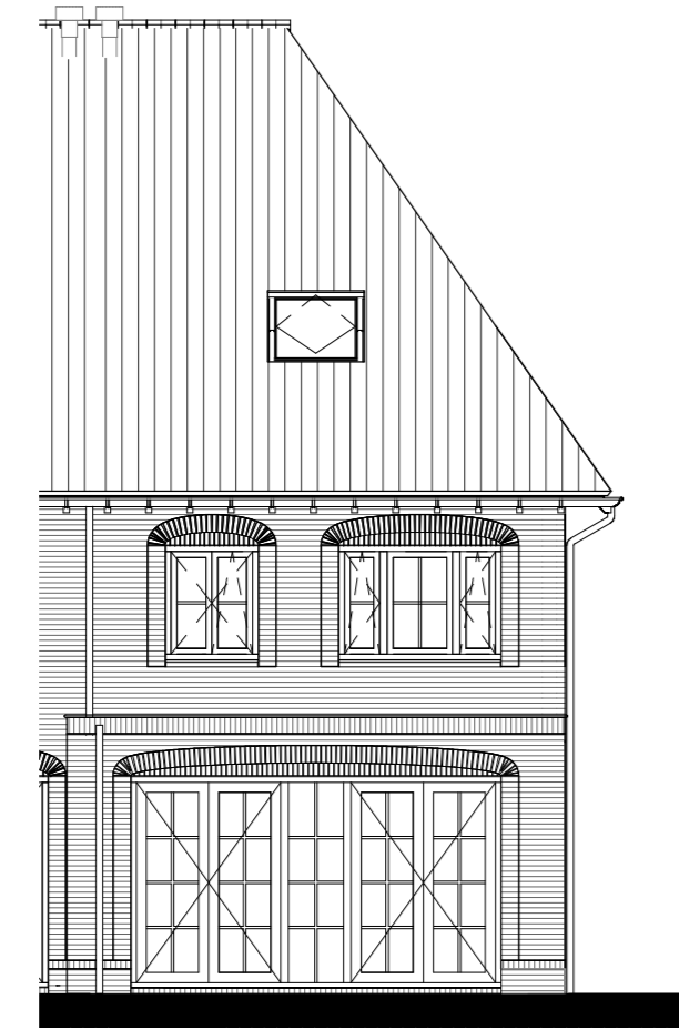
Uitbouw 3200mm getekend: bwnr 23,28 gepegeld: bwnr 24,29
