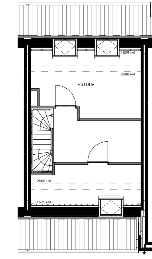
Dakraam voorgevel (verwarmingsopstelling) getekend: bwnr 24 gepegeld: bwnr 28
