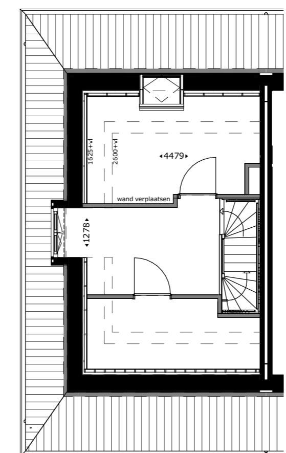
Dakkapel zijgevel (verwarmingsopstelling) getekend: bwnr 29 gepegeld: bwnr 29
