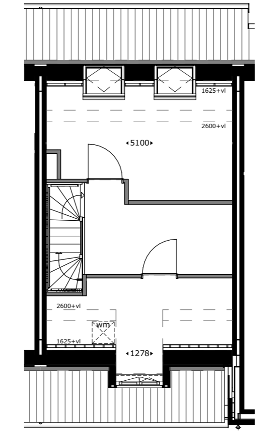
Dakkapel voorgevel (verwarmingsopstelling) getekend: bwnr 24 gepegeld: bwnr 28
