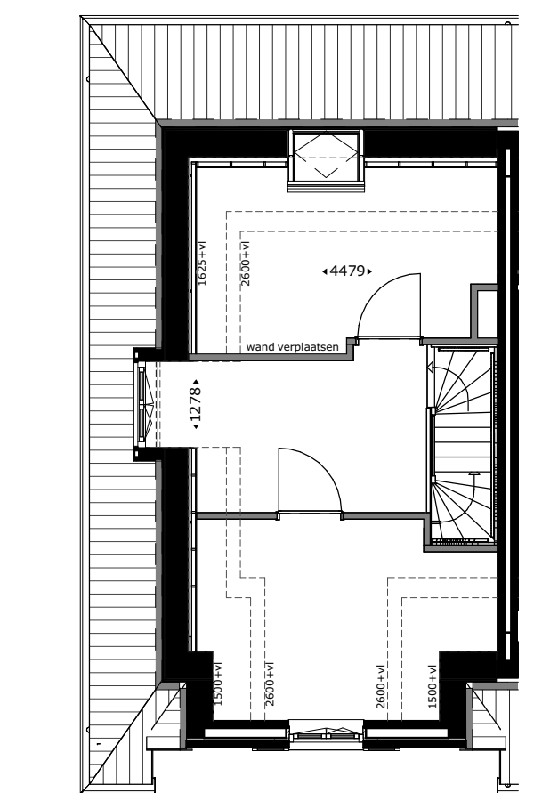
Dakkapel scheringewelf getekend: bwnr 05,11 gespegeld: bwnr 12
