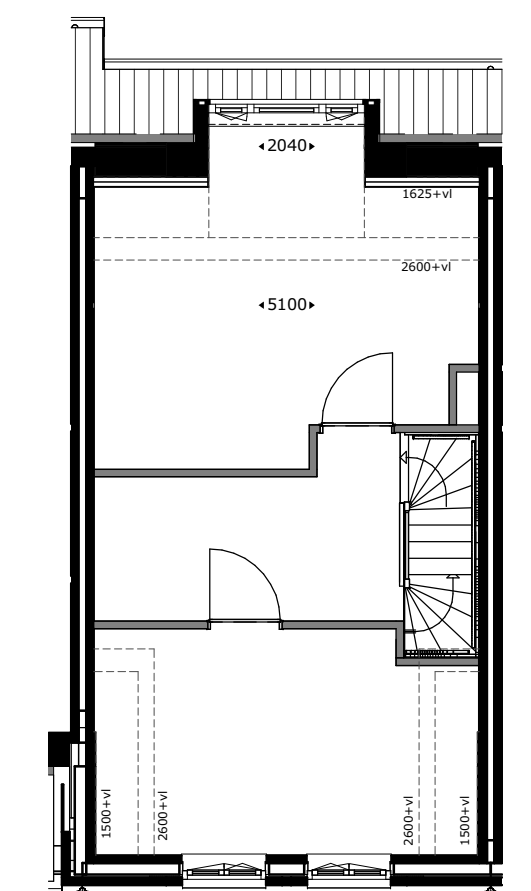
Dakkapel scheringewelf getekend: bwnr 07,09 gespegeld: bwnr 08,10
