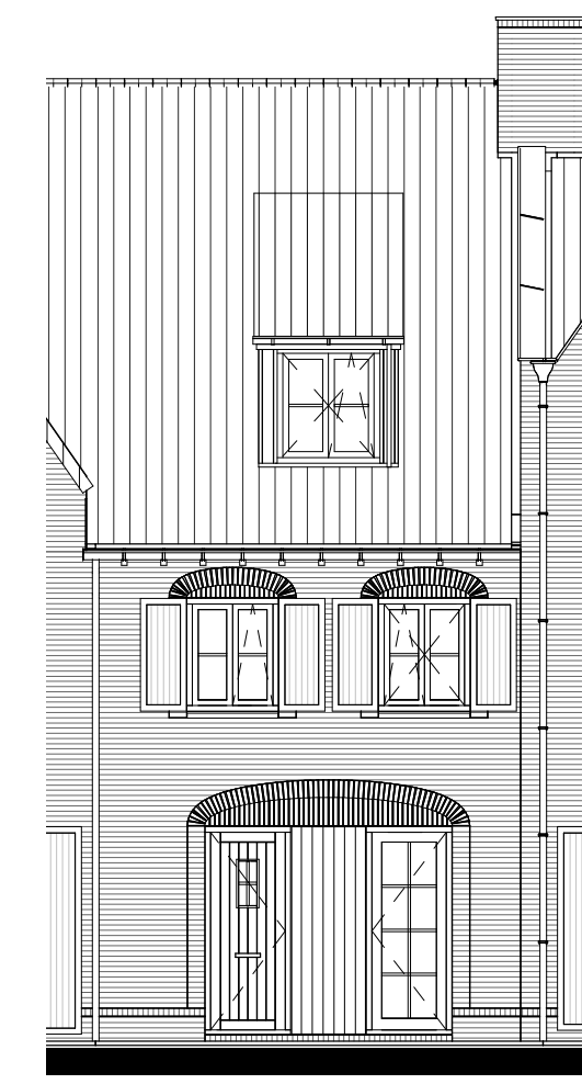
Dakkapel voorgewelf (vergunningsplichtig) getekend: bwnr 06 gespegeld: bwnr 11
