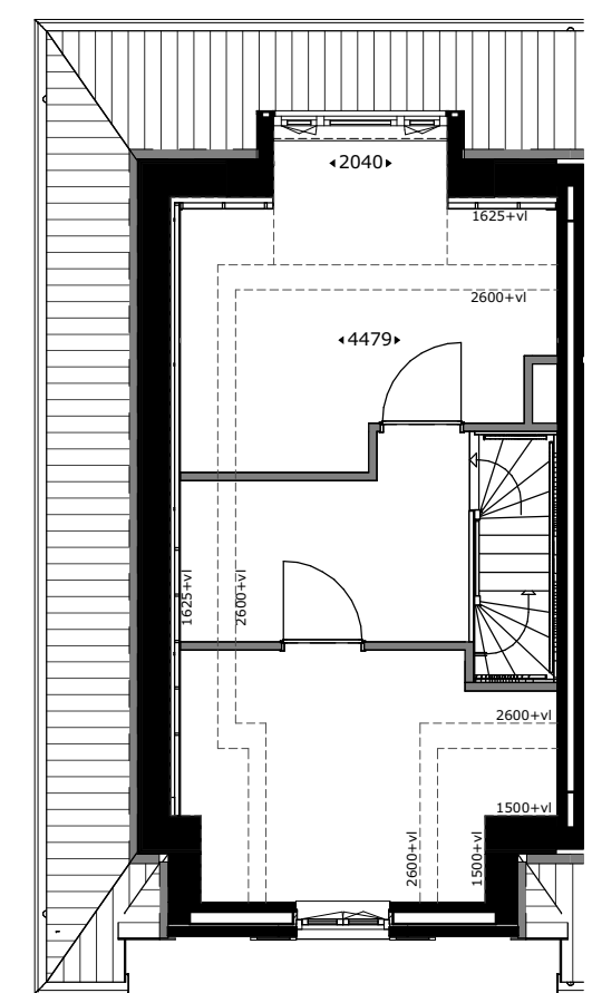
Dakkapel scheringewelf getekend: bwnr 05 gespegeld: bwnr 12
