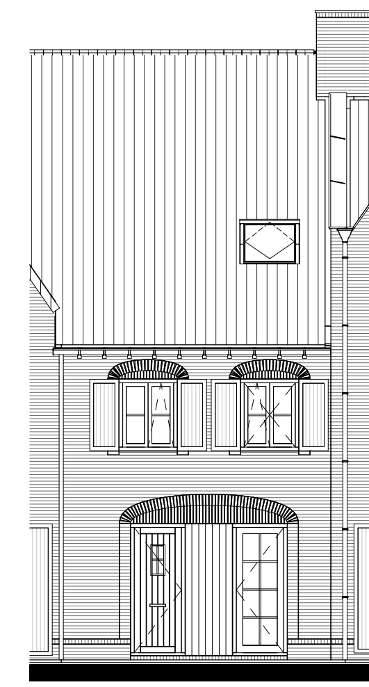
Dakraam voorgewelf (vergunningsplichtig) getekend: bwnr 05 gespegeld: bwnr 11
