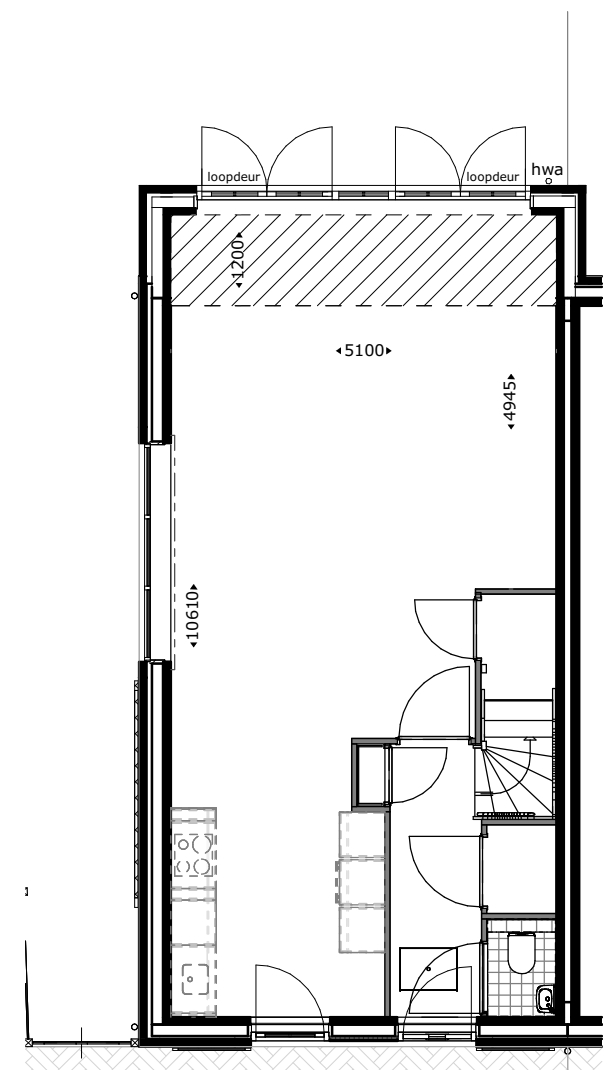
Uitbouw 3200mm getekend: bwnr 05,11 gespegeld: bwnr 06,12
