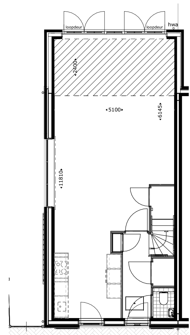
Uitbouw 2400mm getekend: bwnr 05,11 gespegeld: bwnr 06,12
