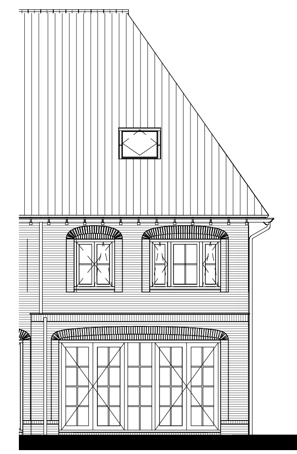
Uitbouw 2400mm getekend: bwnr 05,11 gespegeld: bwnr 06,12
