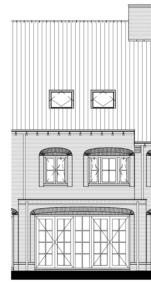
Uitbouw 2400mm getekend: bwnr 07,09 gespegeld: bwnr 08,10
