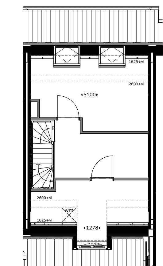
Dakkapel voorgewelf (vergunningsplichtig) getekend: bwnr 06 gespegeld: bwnr 11
