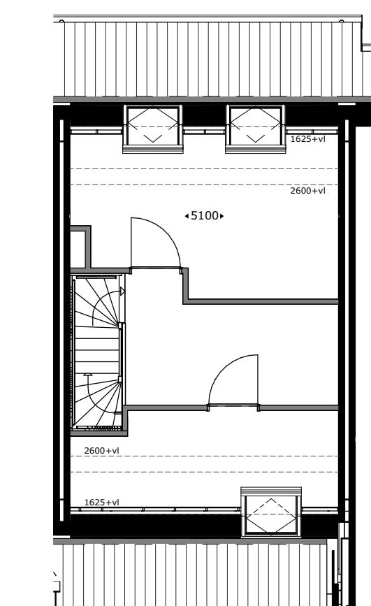
Dakraam voorgewelf (vergunningsplichtig) getekend: bwnr 05 gespegeld: bwnr 11
