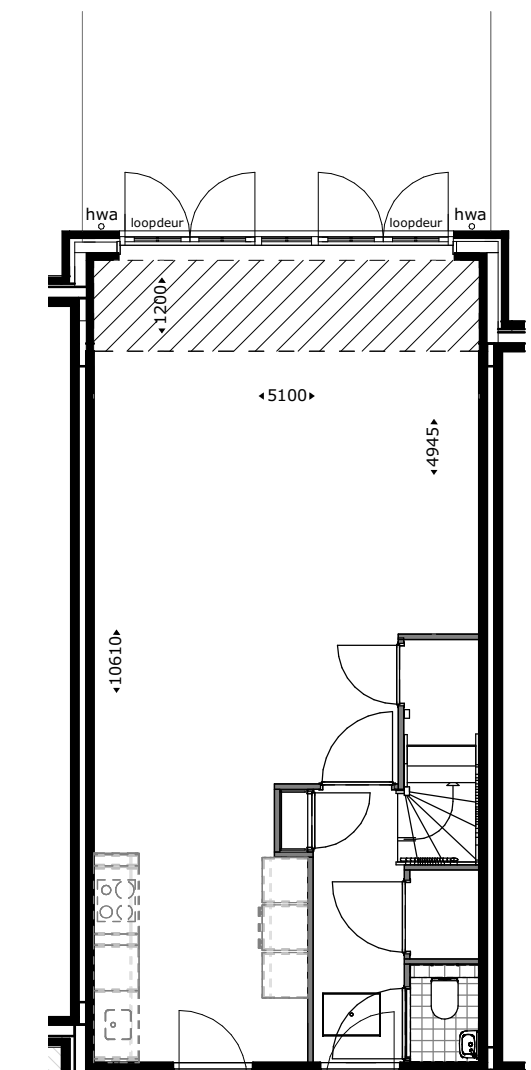
Uitbouw 3200mm getekend: bwnr 07,09 gespegeld: bwnr 08,10
