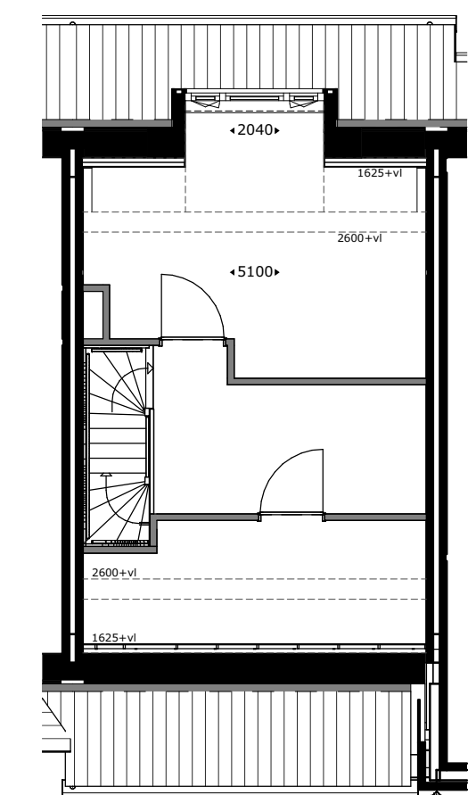
Dakkapel scheringewelf getekend: bwnr 06 gespegeld: bwnr 11
