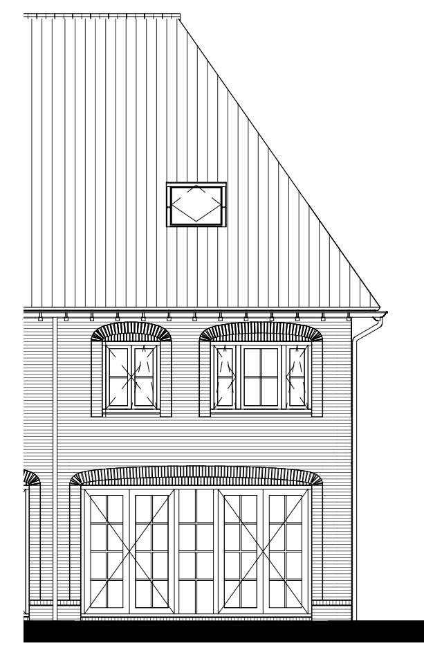
Vergruete pui getekend: bwnr 05,07,09,11 gespegeld: bwnr 06,08,10,12
