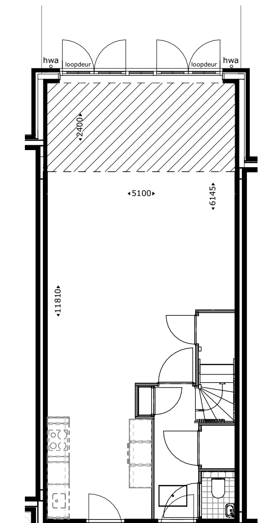
Uitbouw 2400mm getekend: bwnr 07,09 gespegeld: bwnr 08,10
