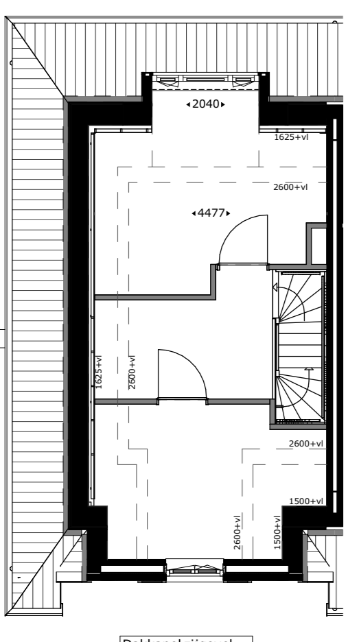
Dakkapel afgewerkt getekend: bwnr 13 gespegeld: bwnr 20
