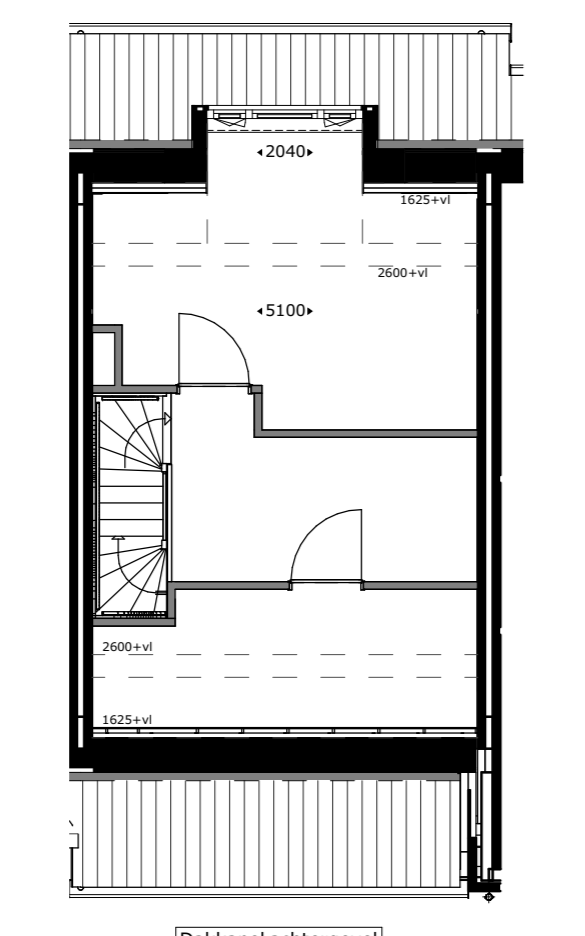
Dakkapel afgewerkt getekend: bwnr 14 gespegeld: bwnr 15
