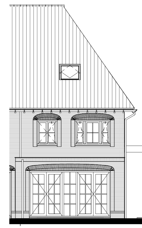
Uitbouw 2400mm getekend: bwnr 13,19 gespegeld: bwnr 14,20
