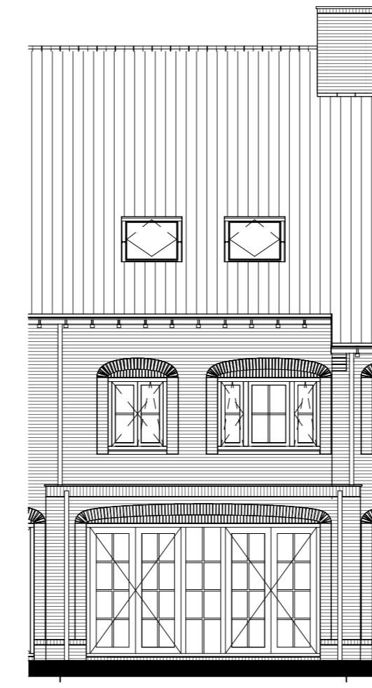
Uitbouw 2400mm getekend: bwnr 15,17 gespegeld: bwnr 16,18
