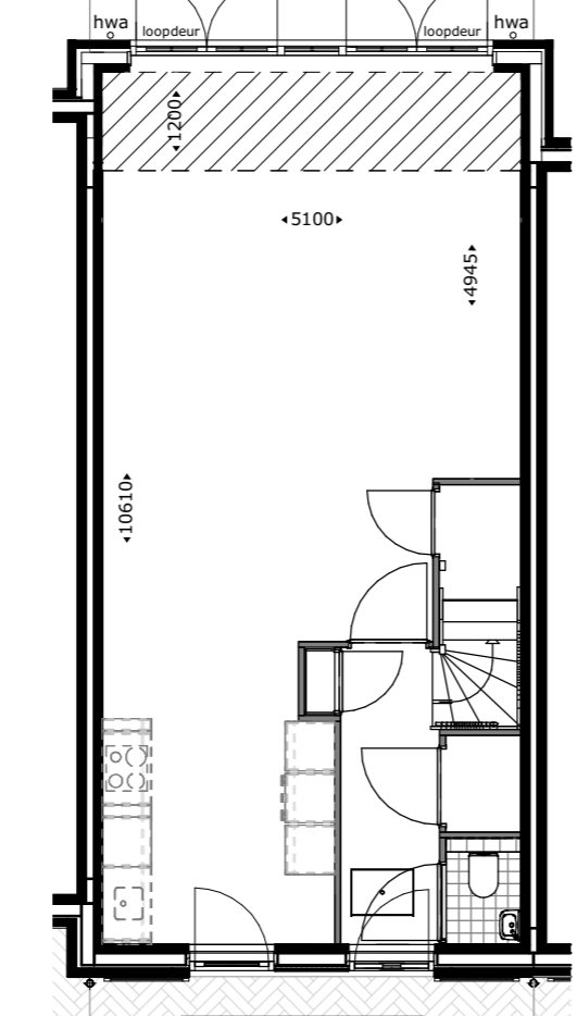
Uitbouw 1200mm getekend: bwnr 15,17 gespegeld: bwnr 16,18
