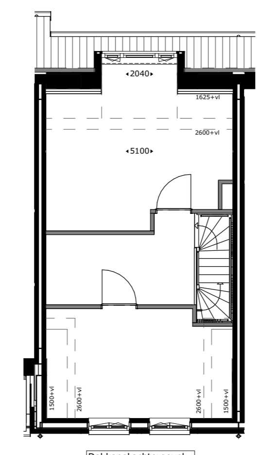
Dakkapel afgewerkt getekend: bwnr 15,17 gespegeld: bwnr 16,18
