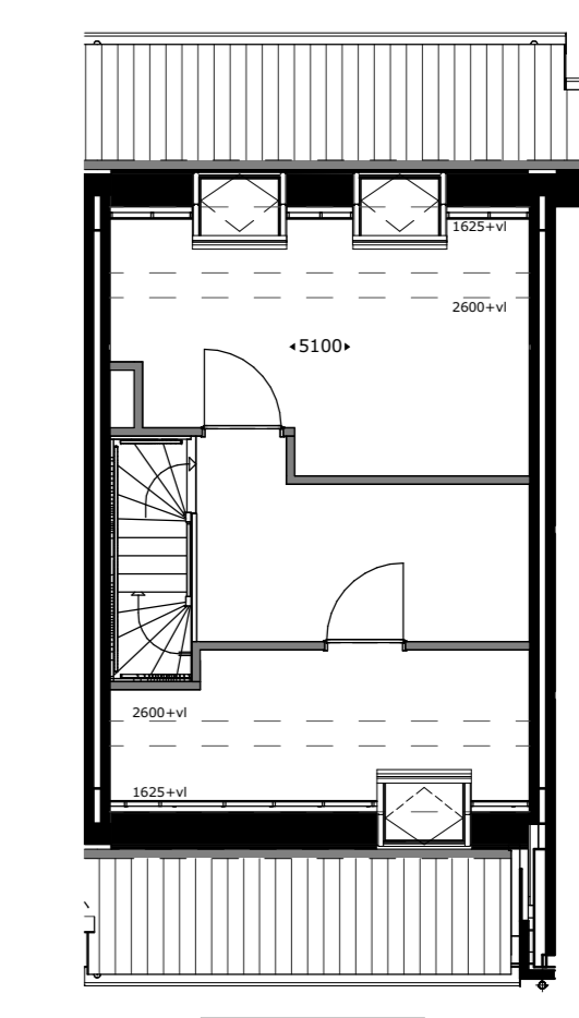
Dakraam voorgoed (verpunningplichtig) getekend: bwnr 14 gespegeld: bwnr 15
