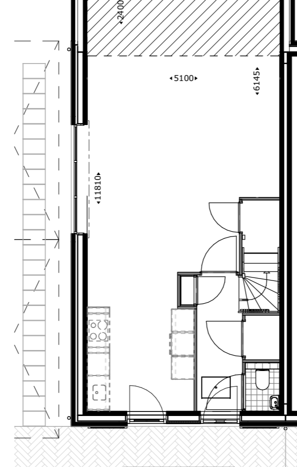
Uitbouw 2400mm getekend: bwnr 13,19 gespegeld: bwnr 14,20
