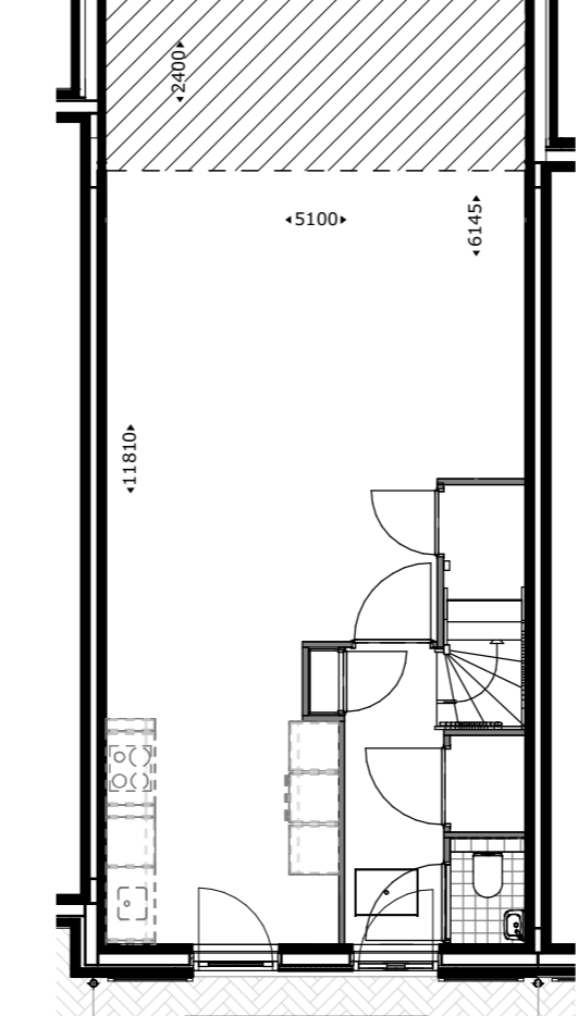
Uitbouw 2400mm getekend: bwnr 15,17 gespegeld: bwnr 16,18
