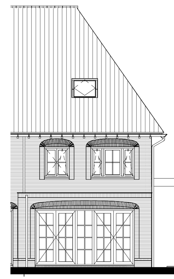
Uitbouw 1200mm getekend: bwnr 13,19 gespegeld: bwnr 14,20
