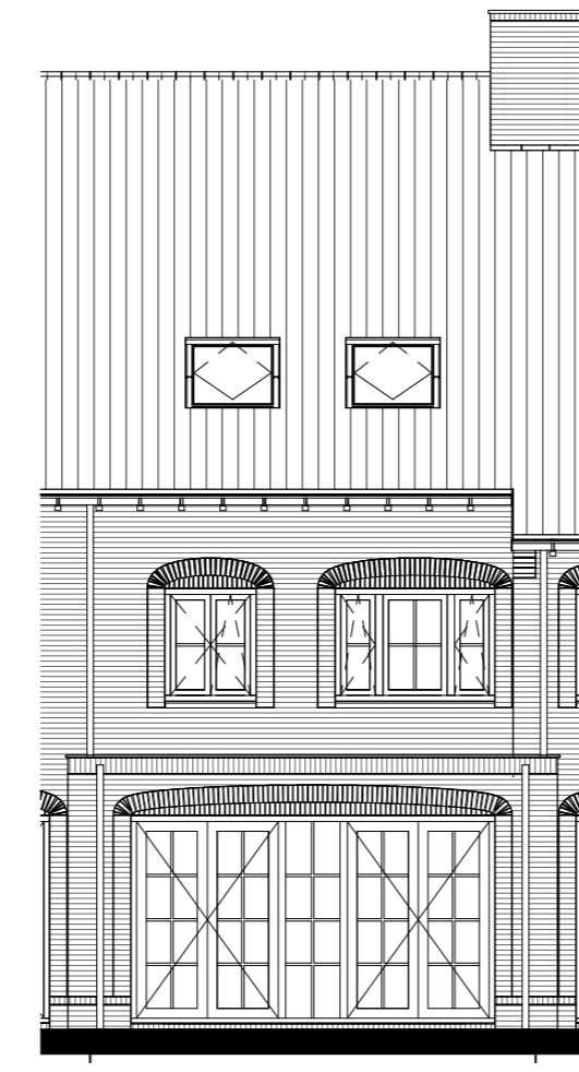
Uitbouw 1200mm getekend: bwnr 15,17 gespegeld: bwnr 16,18
