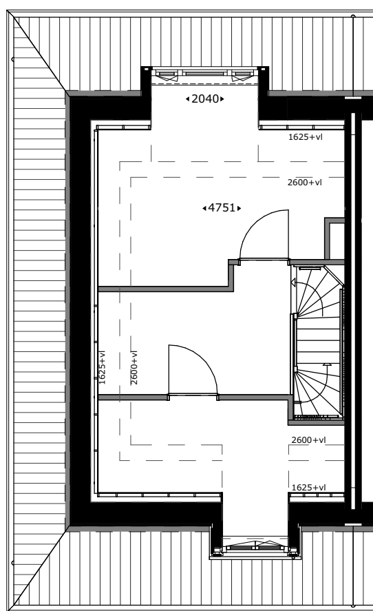
Dakkapel achtergevel getekend : bwnr 32,36,40 gespiegeld : bwnr 33,37,41
