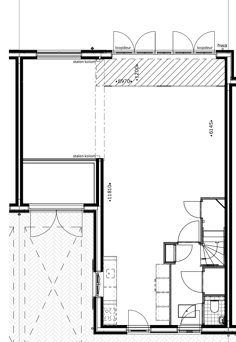
Uitbouw 200mm getekend : bwnr 34,36,38,40,42 gespiegeld : bwnr 33,35,37,39,41,43
