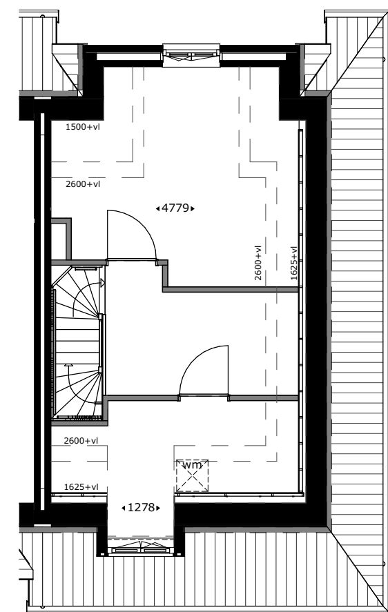
Dakkapel voorgevel (vergunningplichtig) getekend : bwnr 31,35 gespiegeld : bwnr 38,42
