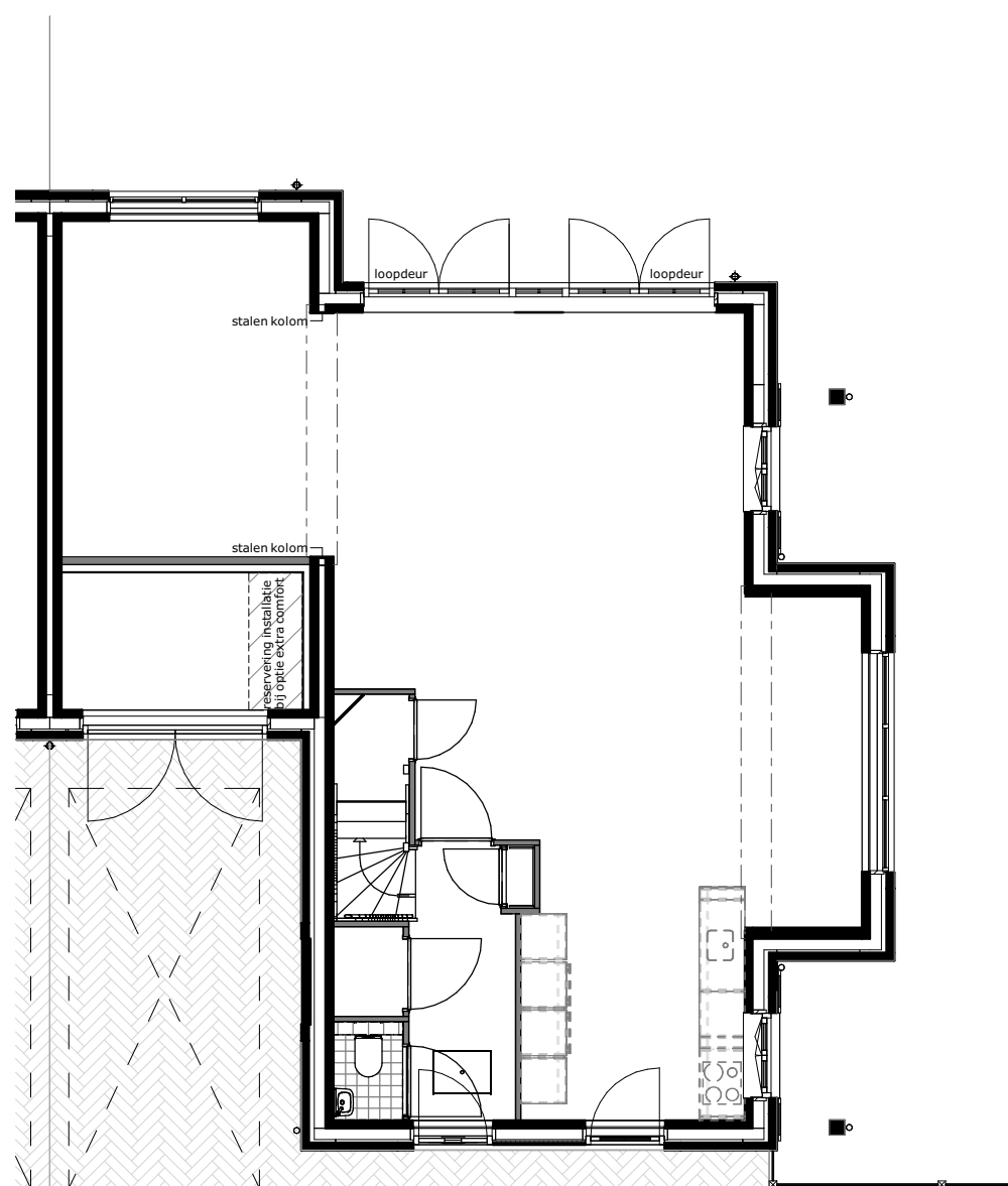
Vergrootte pui getekend : bwnr 44
