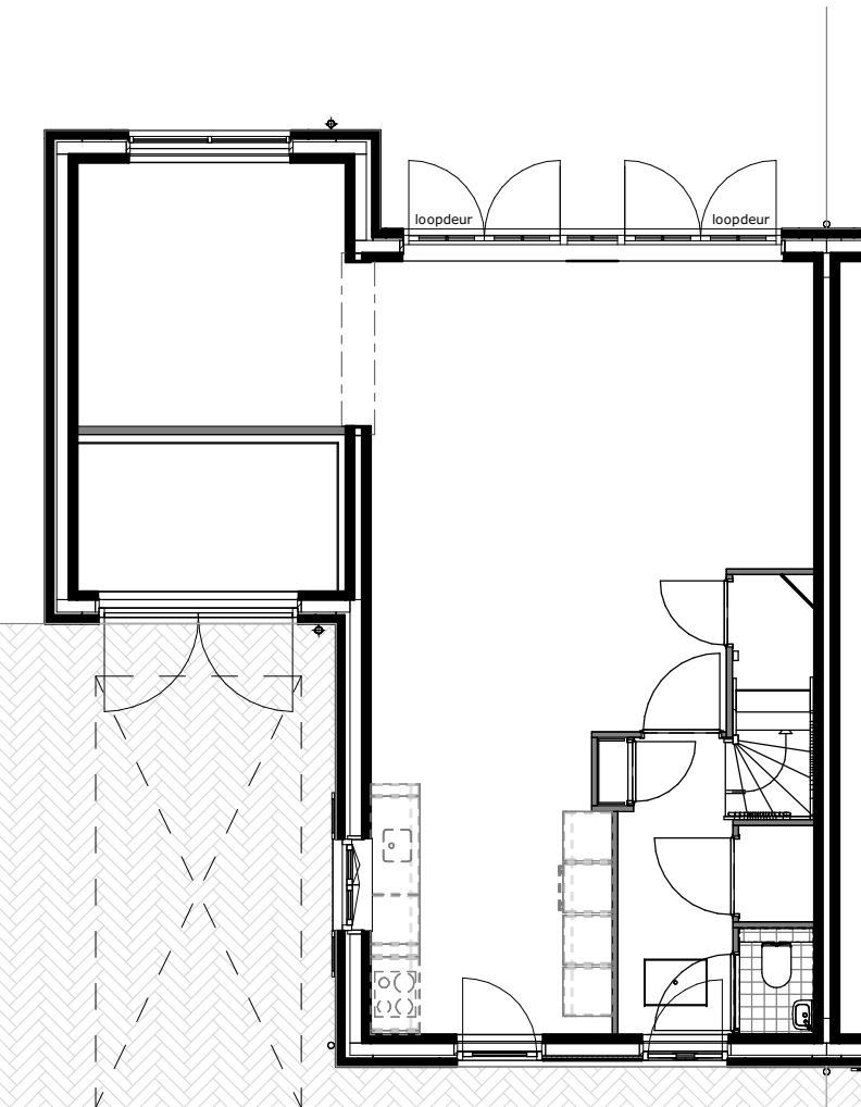
Vergrootte pul getekend : bwnr 30 gespiegeld : bwnr 31
