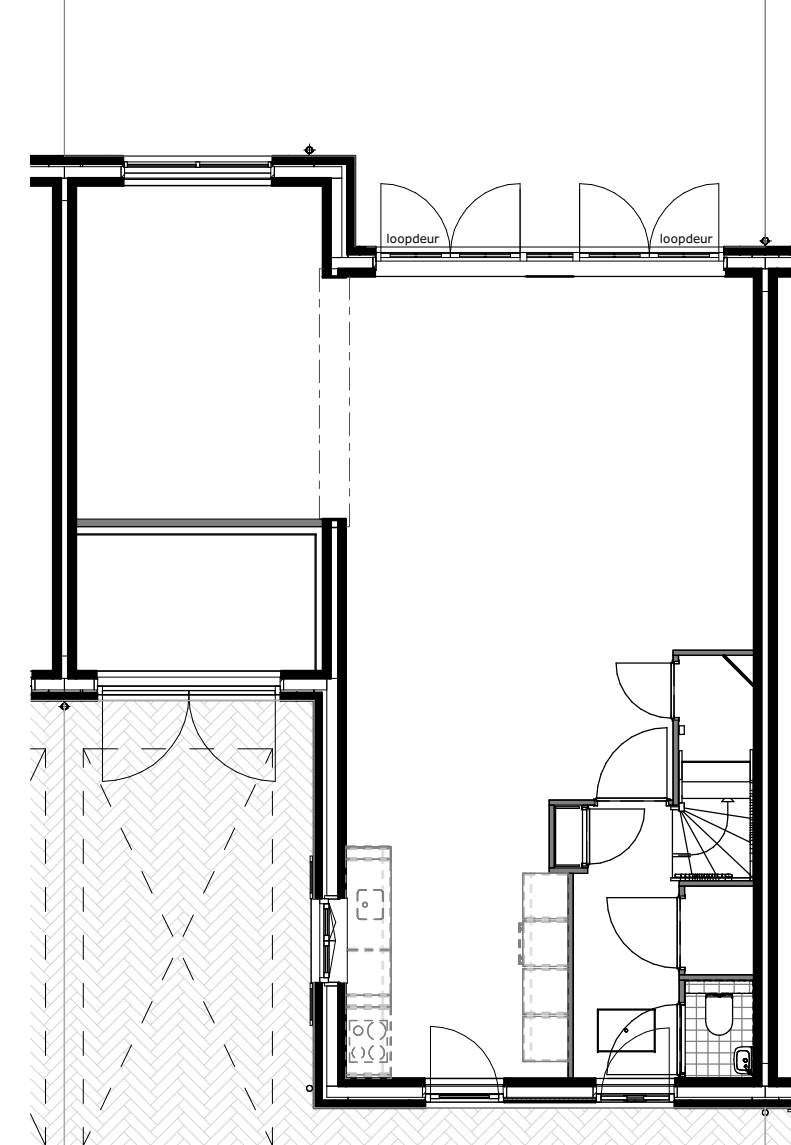
Vergrootte pul getekend : bwnr 34,36,38,40,42 gespiegeld : bwnr 33,35,37,39,41,43
