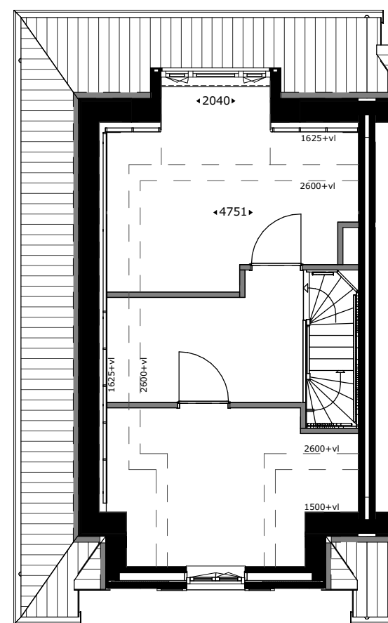
Dakkapel achtergevel getekend : bwnr 30,34 gespiegeld : bwnr 39,43
