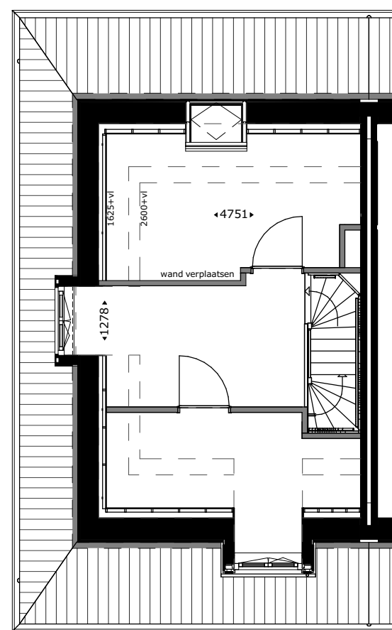
Dakkapel zijgevel (vergunningplichtig) getekend : bwnr 32,36,40 gespiegeld : bwnr 33,37,41
