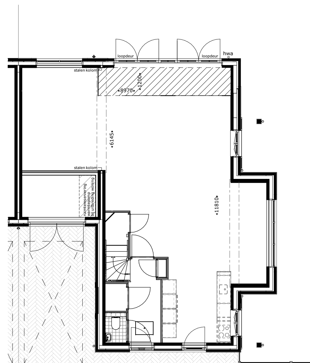
Uitbouw 1200mm. getekend : bwnr 44
