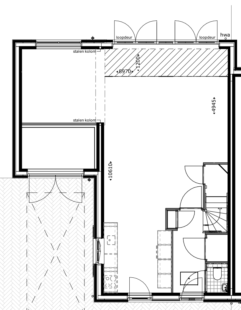
Uitbouw 200mm getekend : bwnr 30 gespiegeld : bwnr 31
