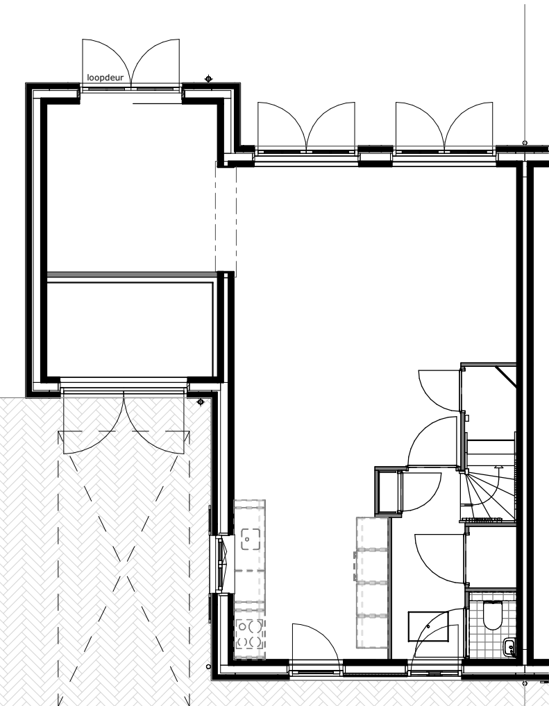
Houten kozijn in turkijamer getekend : bwnr 20 gespiegeld : bwnr 31
